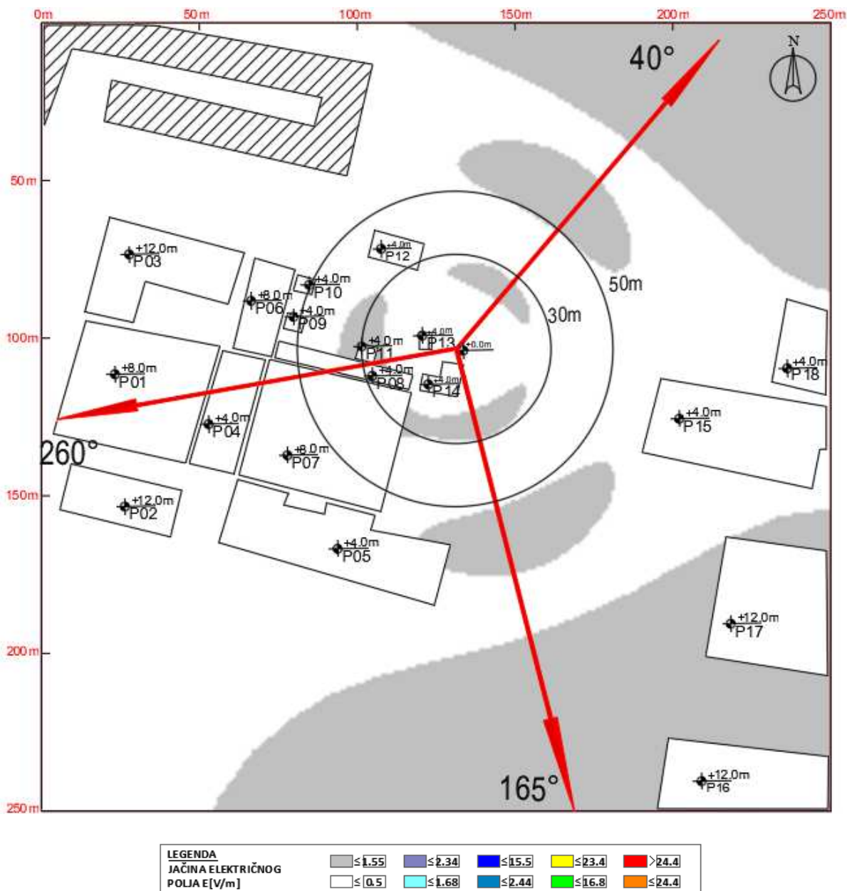
Slika 4.9 Maksimalna proračunata vrednost električnog polja na nivou tla u slučaju rada sistema GSM900 operatora Telekom iznosi: 1.26 V/m
