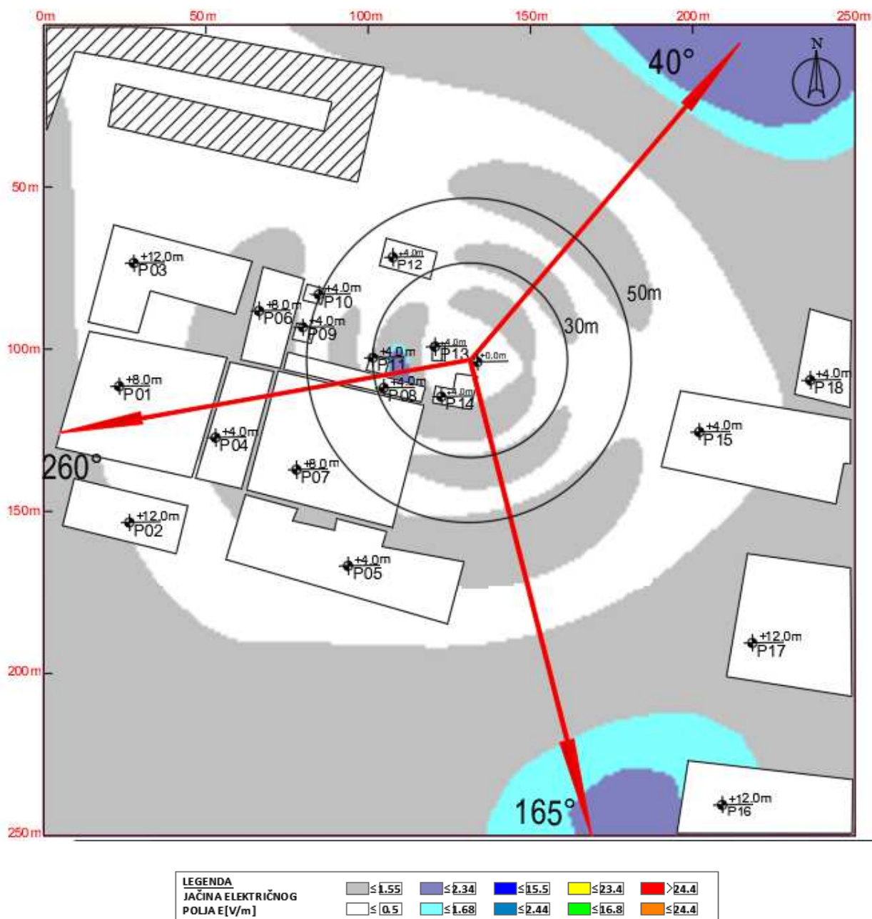
Slika 4.12 Maksimalna proračunata vrednost električnog polja na nivou tla u slučaju rada sistema LTE800 operatora Telekom iznosi: 2.05 V/m
