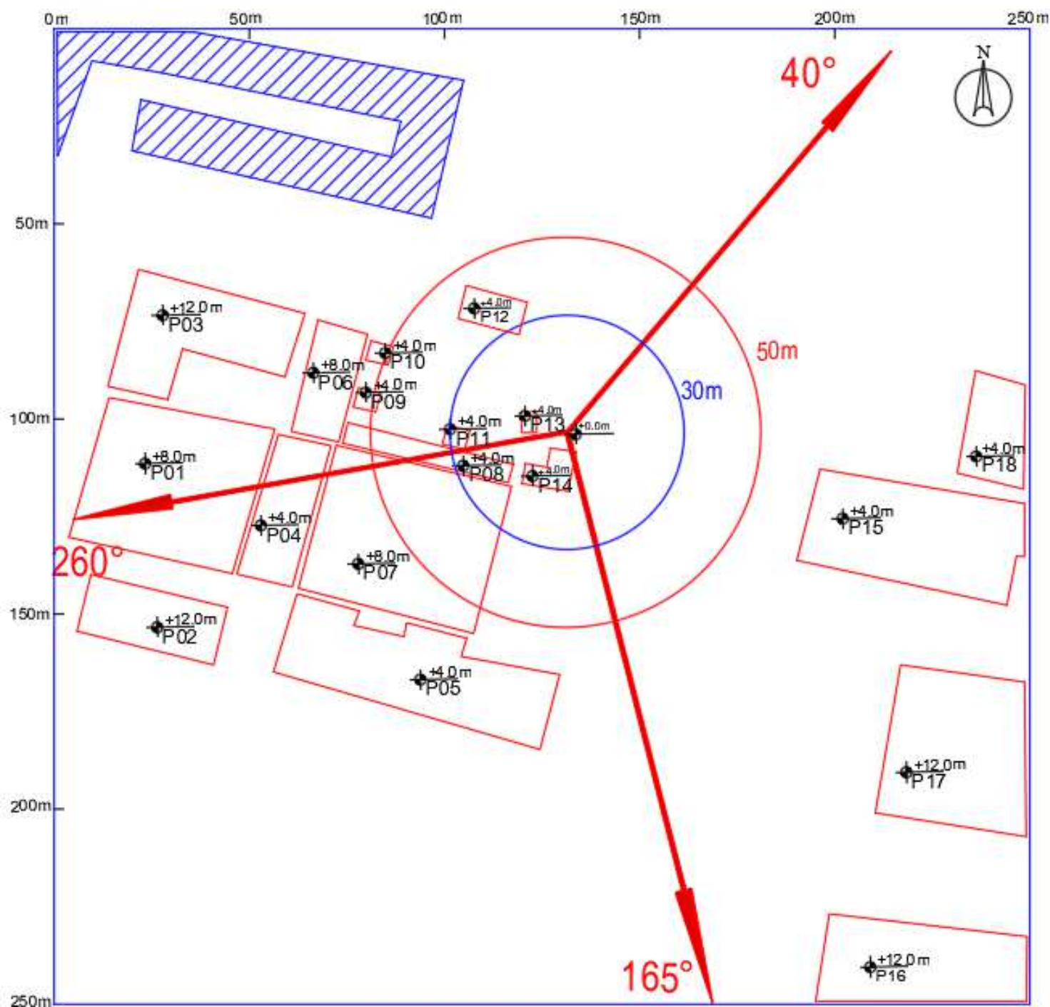
Slika 2.2 Dijagram objekata u okruženju radio bazne stanice „BG - Televizija FOX“ - BG268/BGU268/BGL268/BGO268/BGJ268
