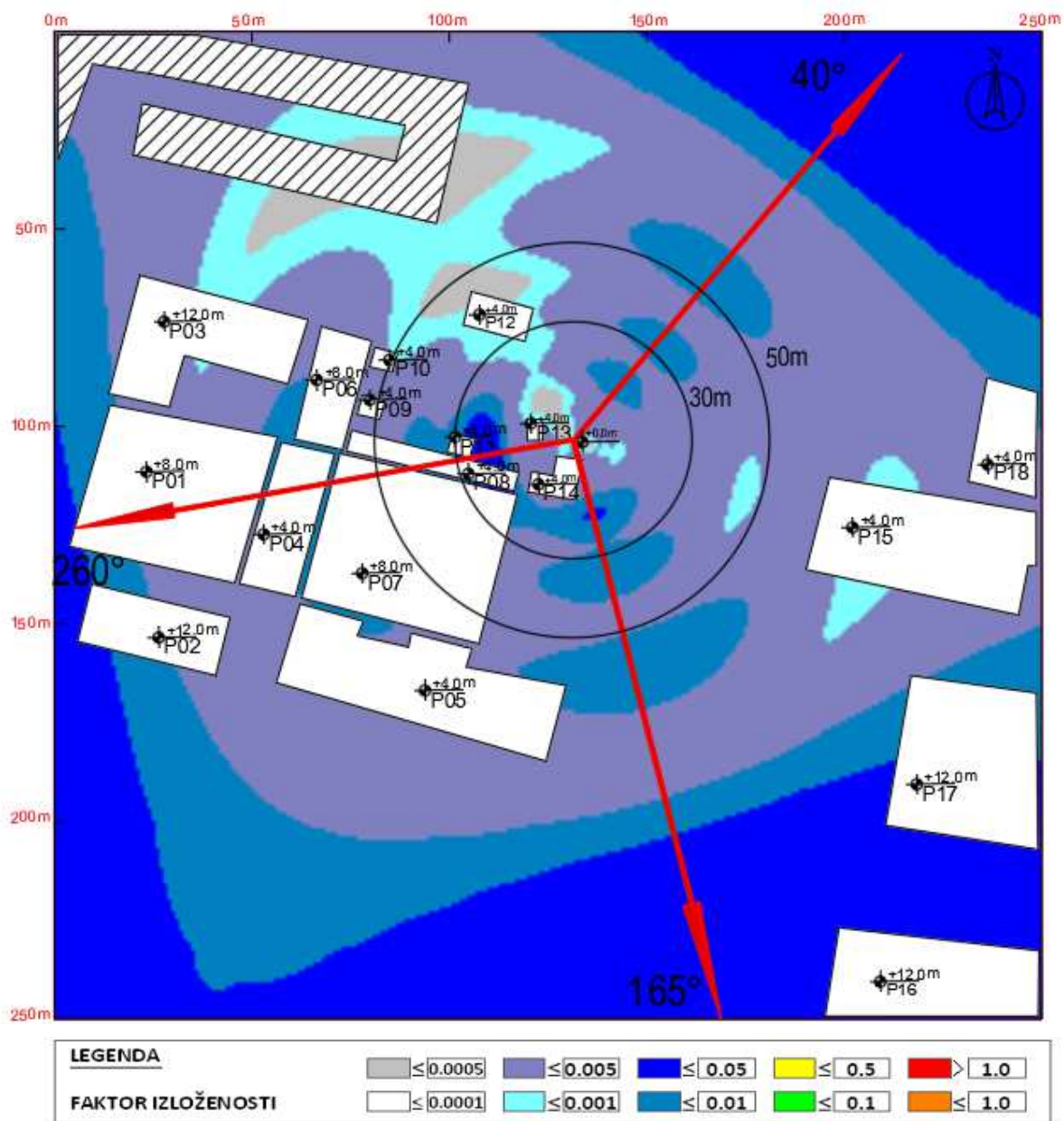
Slika 4.16 Maksimalna proračunata vrednost ukupnog faktora izloženosti na nivou tla u slučaju rada svih sistema na predmetnoj lokaciji operatora Telekom i A1 SRBIJA mobile iznosi: 0.0297 .
