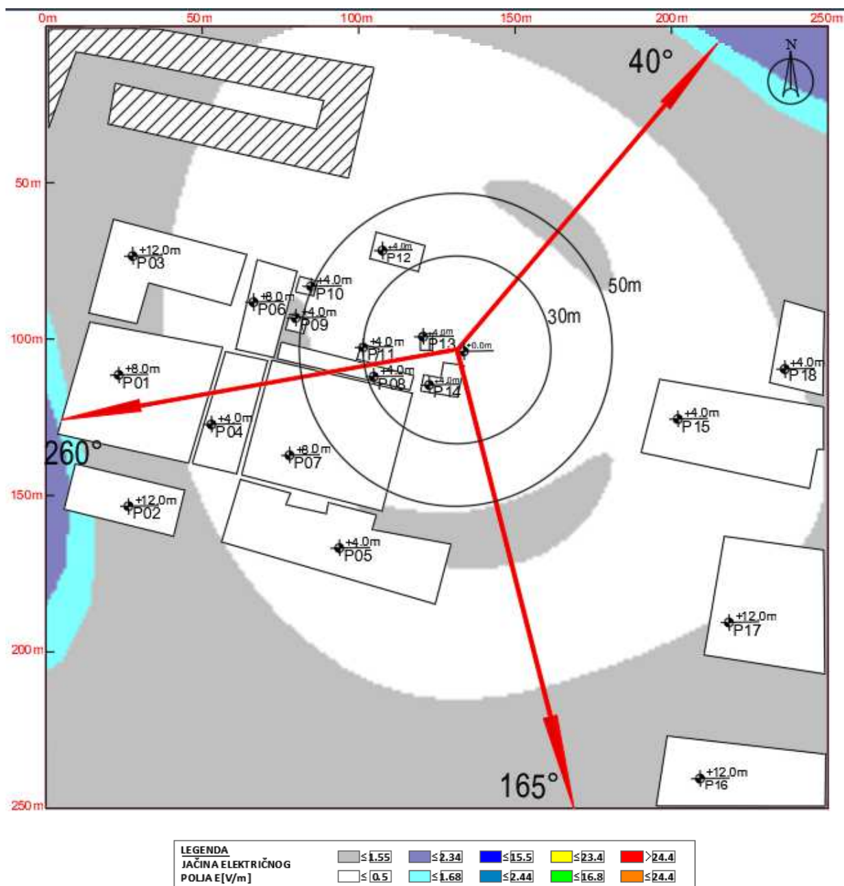
Slika 4.11 Maksimalna proračunata vrednost električnog polja na nivou tla u slučaju rada sistema LTE1800 operatora Telekom iznosi: 1.85 V/m
