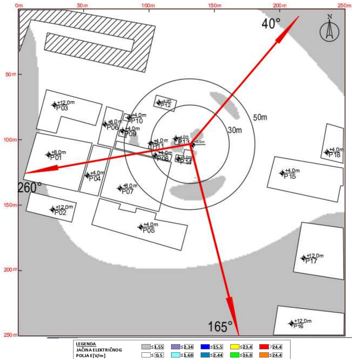
Slika 4.10 Maksimalna proračunata vrednost električnog polja na nivou tla u slučaju rada sistema UMTS2100 operatora Telekom iznosi: 1.27 V/m
