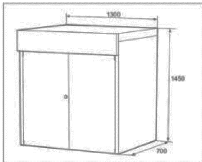
Slika 8.2 Dimenzije RBS6101
