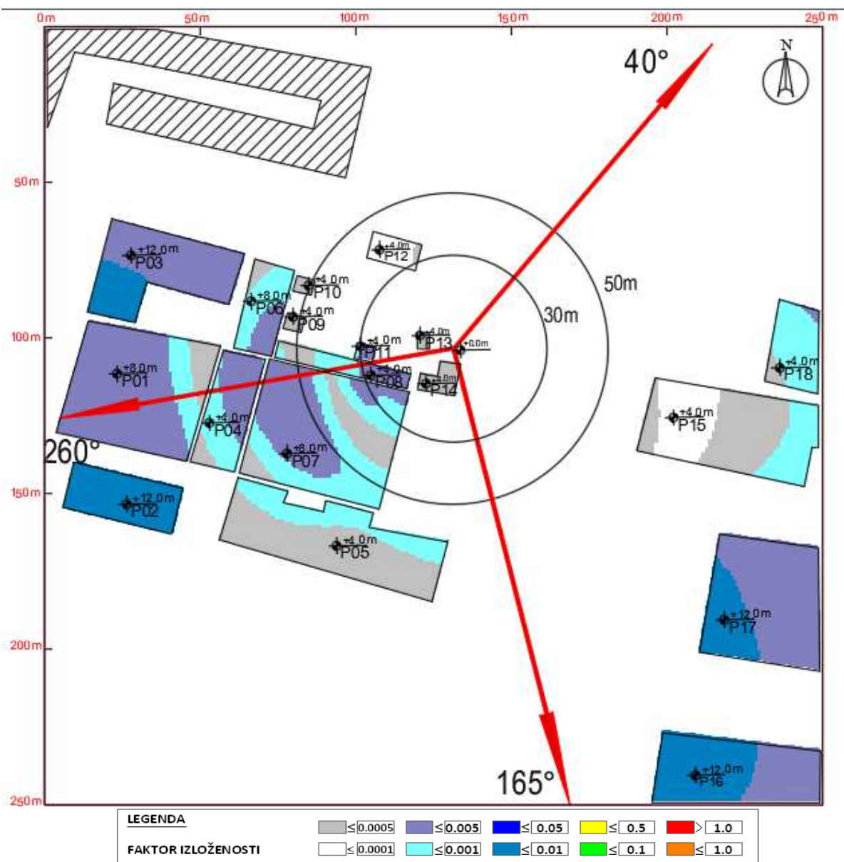
Slika 4.6 Rezultati proračuna faktora izloženosti u objektima na najizloženijim spratovima za slučaj rada sistema GSM900/UMTS2100/LTE1800/LTE800/LTE2100 operatora Telekom Srbija
