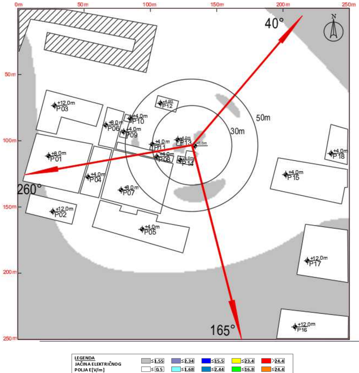
Slika 4.13 Maksimalna proračunata vrednost električnog polja na nivou tla u slučaju rada sistema LTE2100 operatora Telekom iznosi: 1.21 V/m
