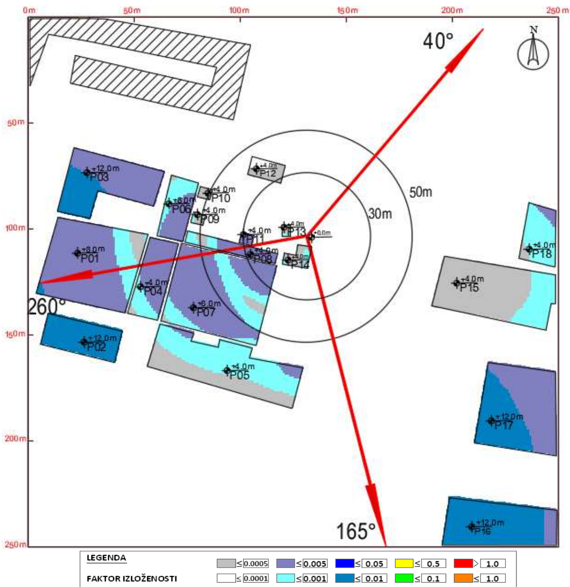
Slika 4.8 Rezultati proračuna faktora izloženosti u objektima na najizloženijim spratovima za slučaj rada svih sistema operatora Telekom i A1
