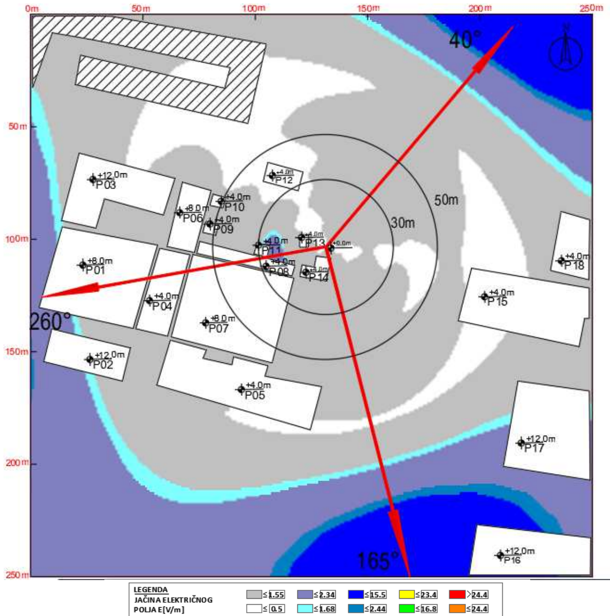
Slika 4.14 Maksimalna proračunata vrednost električnog polja na nivou tla u slučaju rada svih sistema na predmetnoj lokaciji operatora Telekom iznosi: 3.12 V/m .
