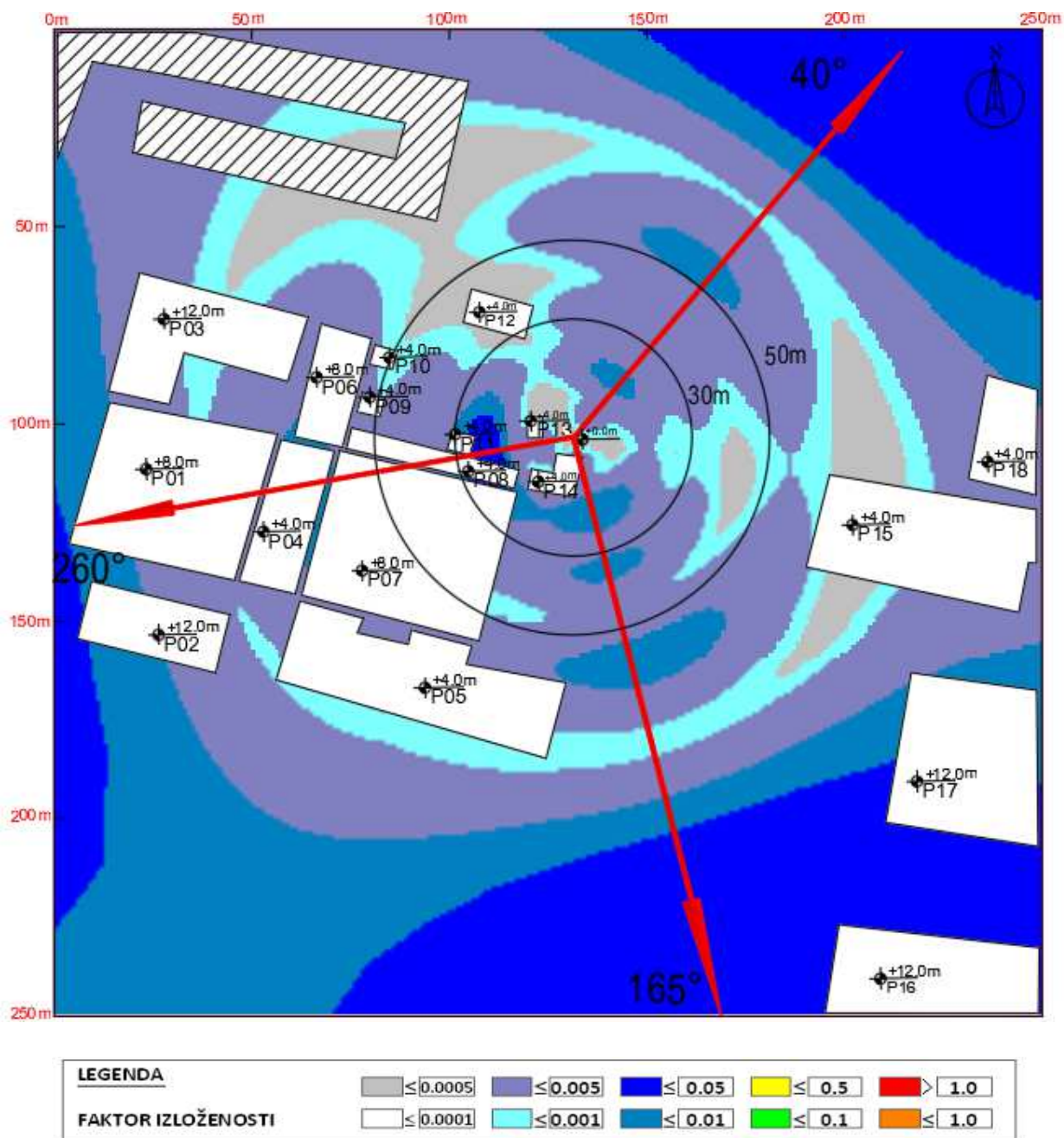
Slika 4.15 Maksimalna proračunata vrednost ukupnog faktora izloženosti na nivou tla u slučaju rada svih sistema na predmetnoj lokaciji operatora Telekom iznosi: 0.0280 .
