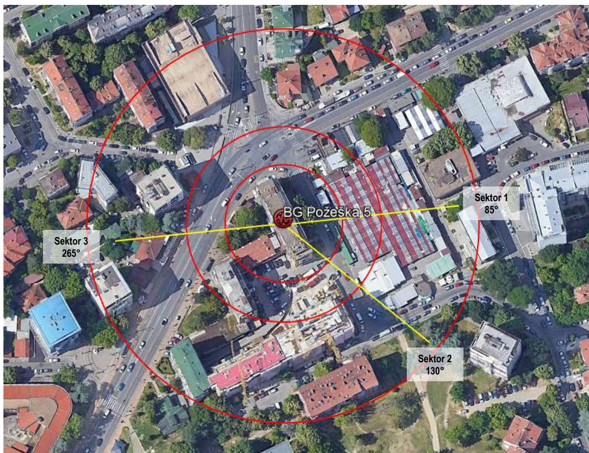
Slika 2.7 Pravci zračenja antenskih sistema predmetne bazne stanice – nakon rekonstrukcije 2.sektora
