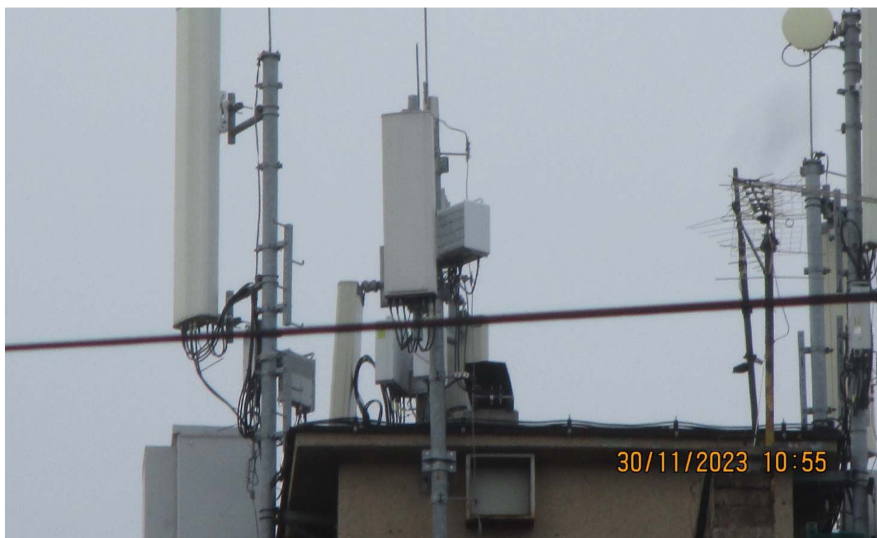
Slika 5: Prikaz antene i radio modula sektora 1
