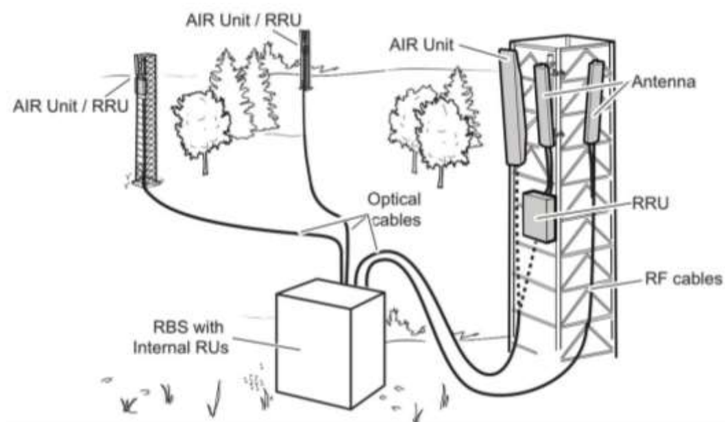
Slika 3.1 Princip konfigurisanja RBS
