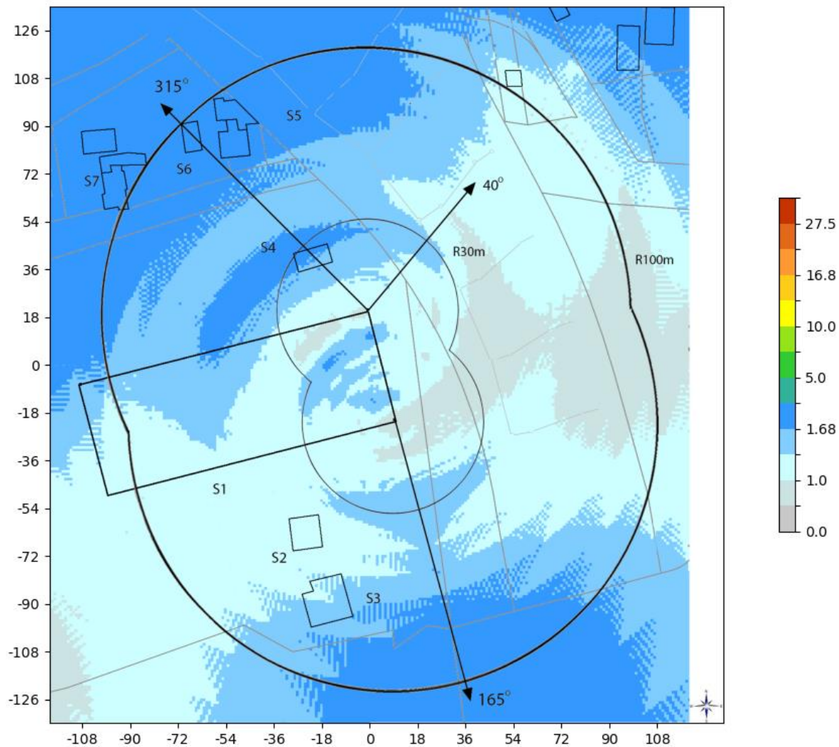
Slika 6.17. Rezultati proračuna jačine električnog polja na tlu, za slučaj kada sve stanice svih operatora rade sa maks. kapacitetom.
