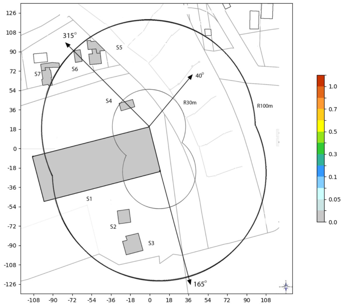
Slika 6.7. Rezultati proračuna faktora izlaganja unutar objekata, kada svi sistemi operatora MTS na lokaciji rade sa maksimalnim kapacitetom.
