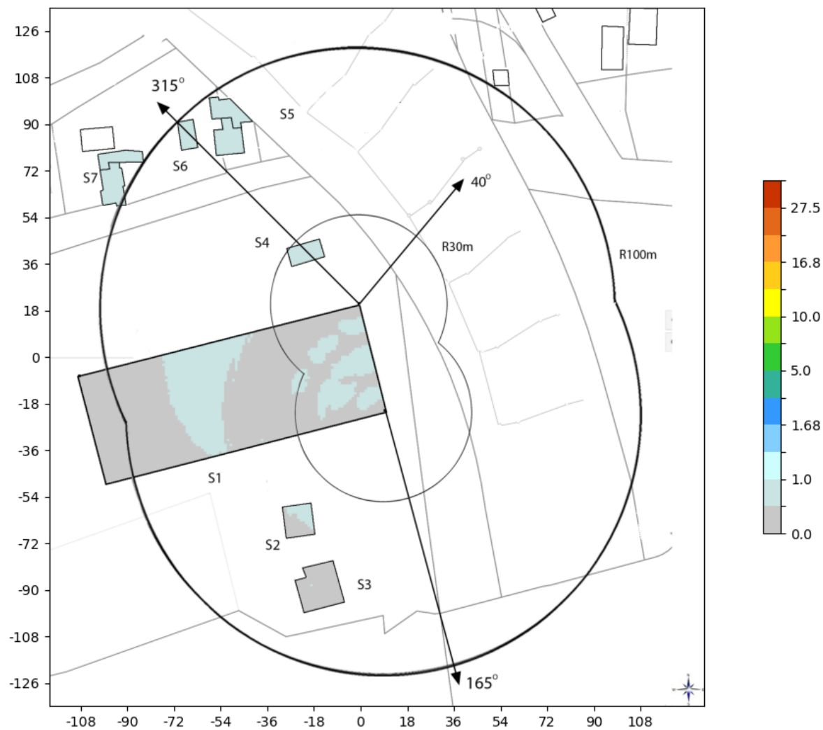
Slika 6.3. Rezultati proračuna jačine električnog polja unutar objekata, kada GSM bazna stanica operatora MTS radi sa maks. kapacitetom.
