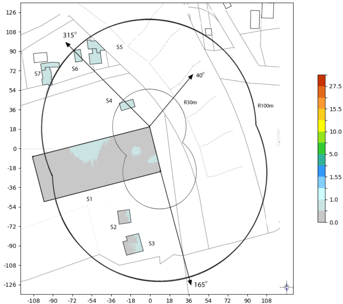
Slika 6.1: Rezultati proračuna jačine električnog polja unutar objekata, kada LTE800 bazna stanica operatora MTS radi sa maksimalnim kapacitetom.
