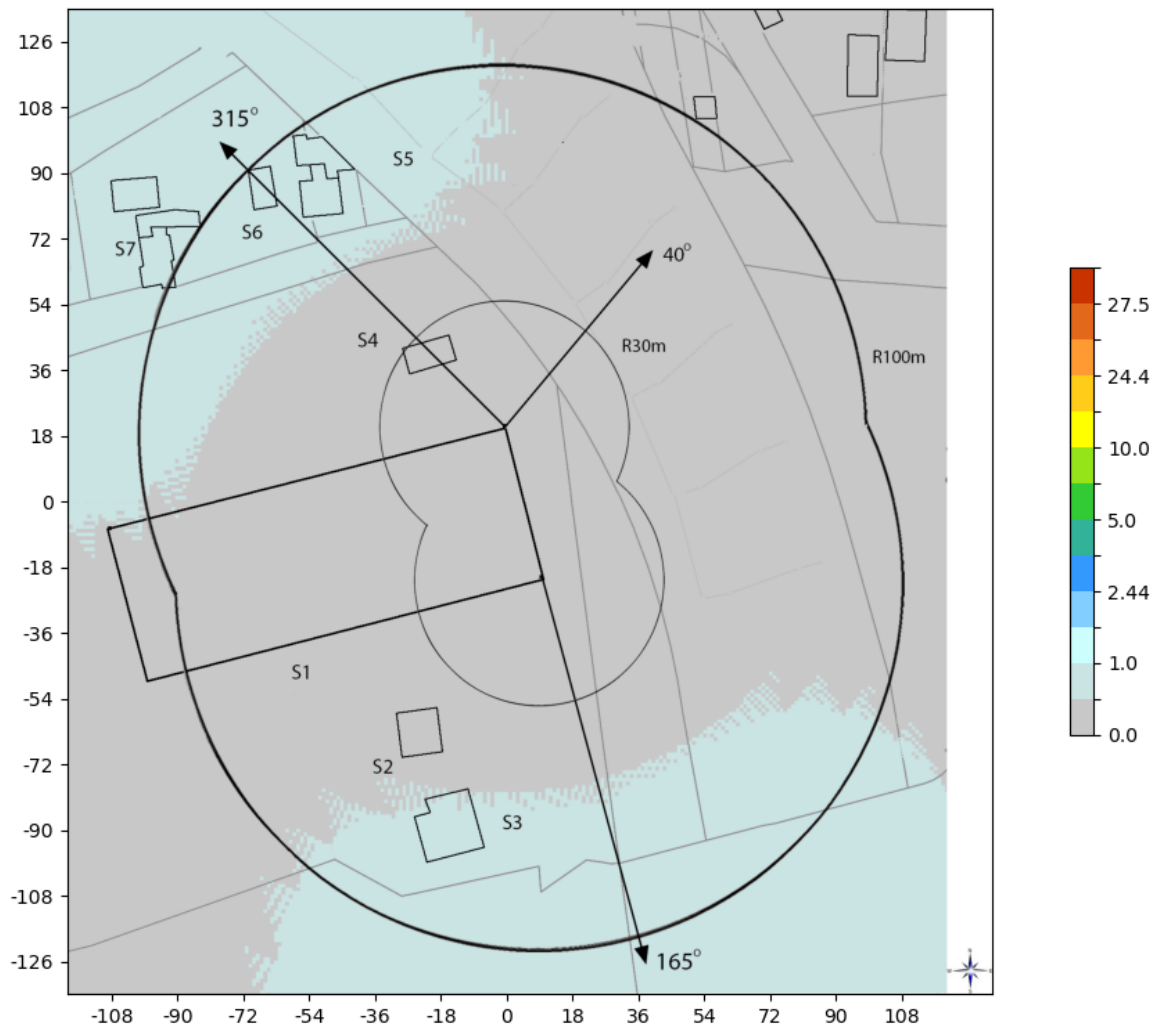
Slika 6.13. Rezultati proračuna jačine električnog polja na tlu, za slučaj kada LTE2100 bazna stanica operatora MTS radi sa maks. kapacitetom.
