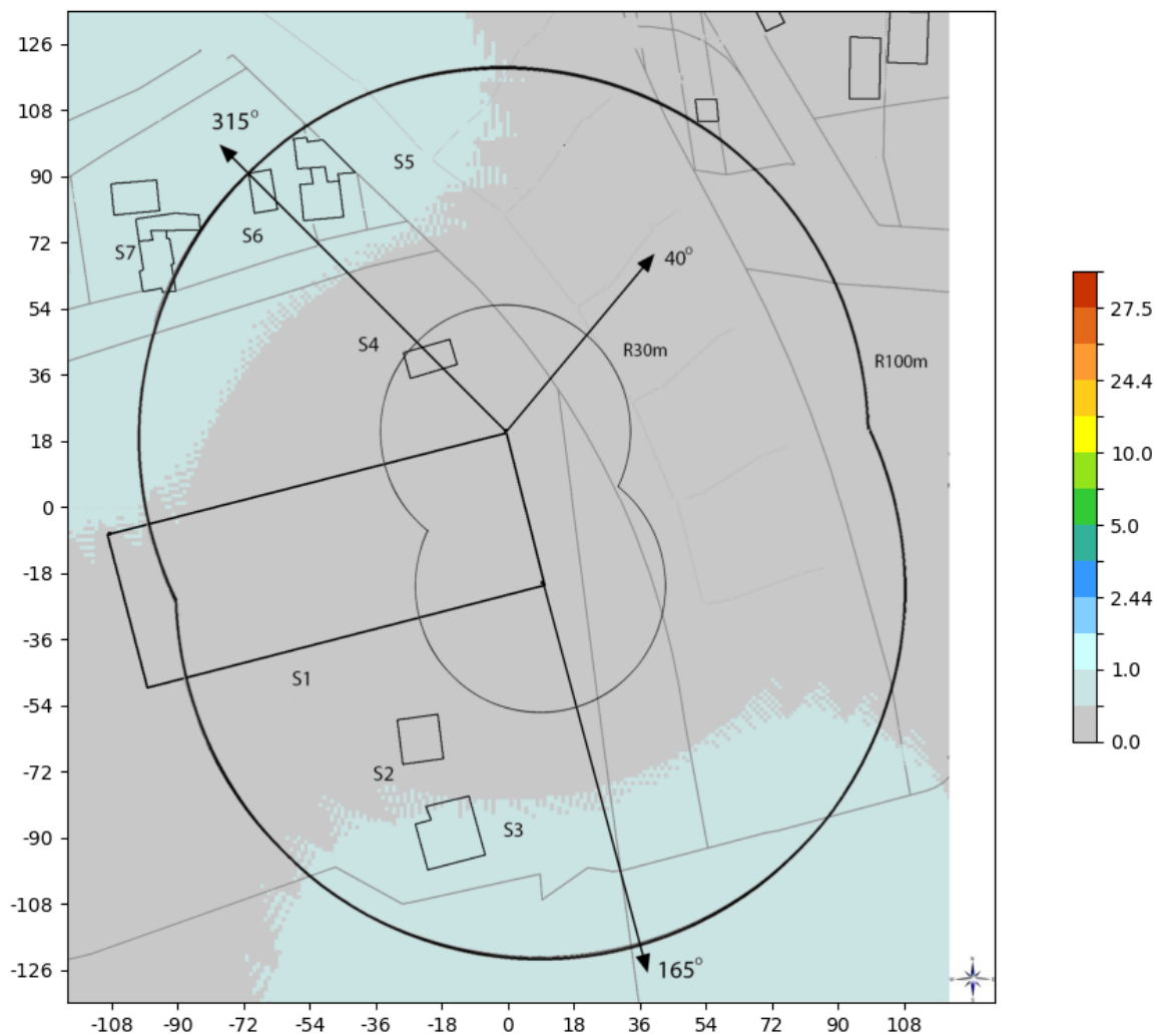
Slika 6.14. Rezultati proračuna jačine električnog polja na tlu, za slučaj kada UMTS2100 bazna stanica operatora MTS radi sa maks. kapacitetom.
