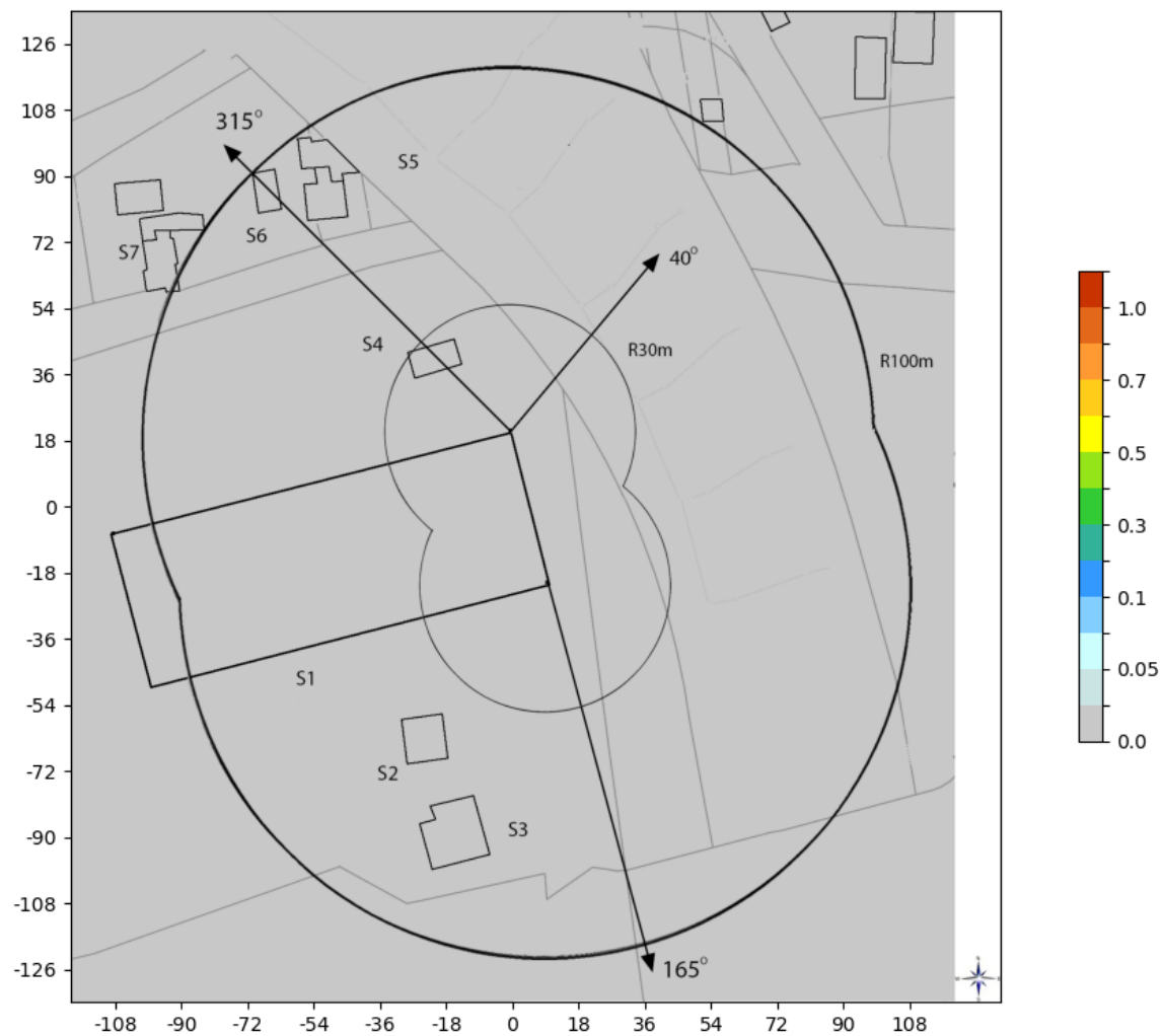
Slika 6.16: Rezultati proračuna faktora izlaganja na tlu, za slučaj kada svi sistemi operatora MTS na lokaciji rade sa maksimalnim kapacitetom
