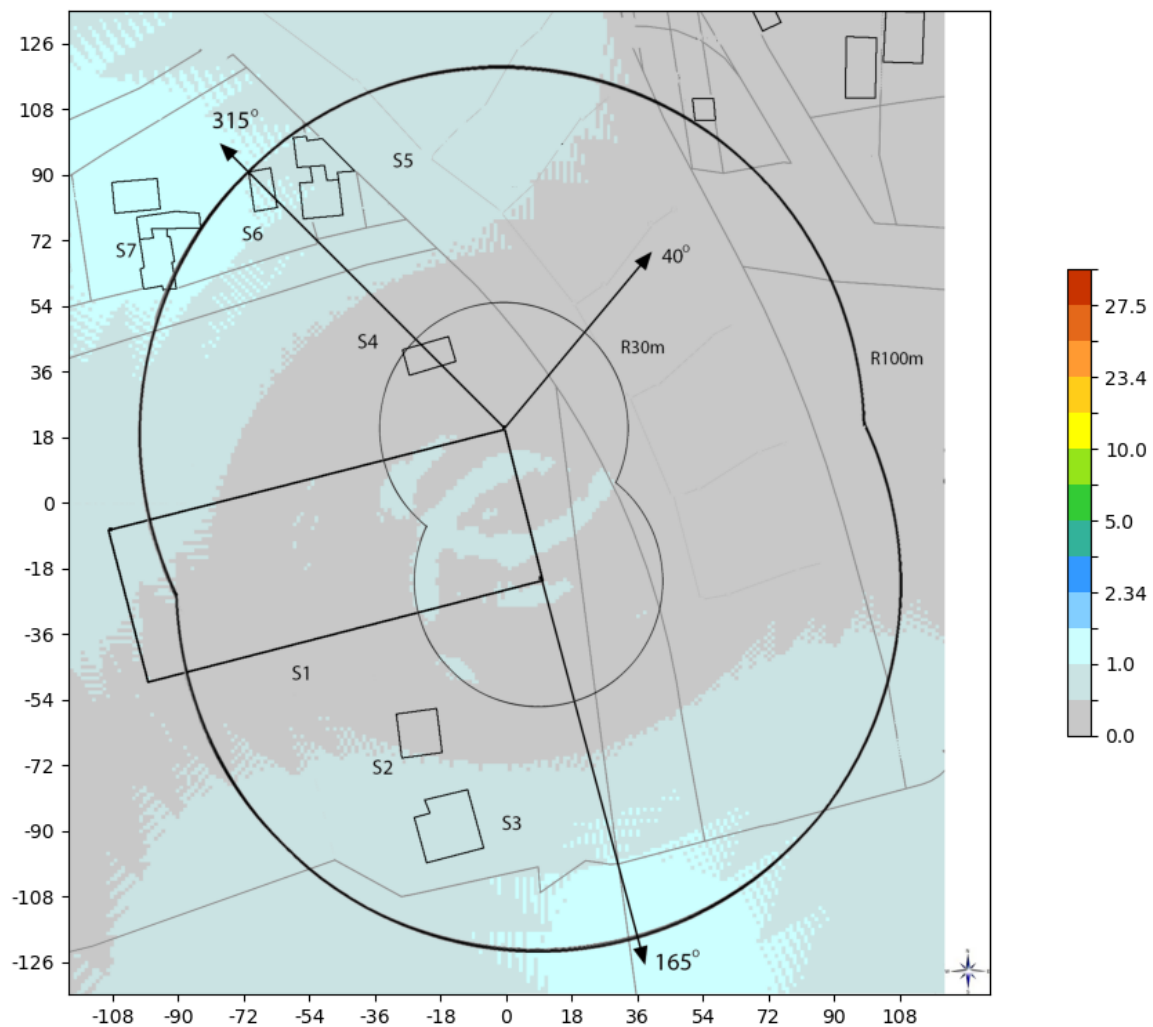
Slika 6.11. Rezultati proračuna jačine električnog polja na tlu, za slučaj kada LTE1800 bazna stanica operatora MTS radi sa maks. kapacitetom.
