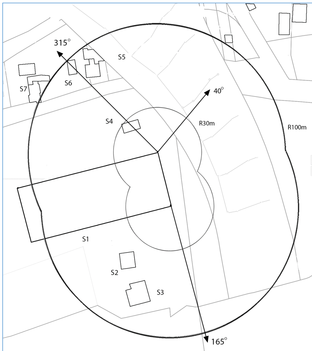
Slika 2.3 Dispozicija objekata u okruženju bazne stanice u krugu 100m od izvora
