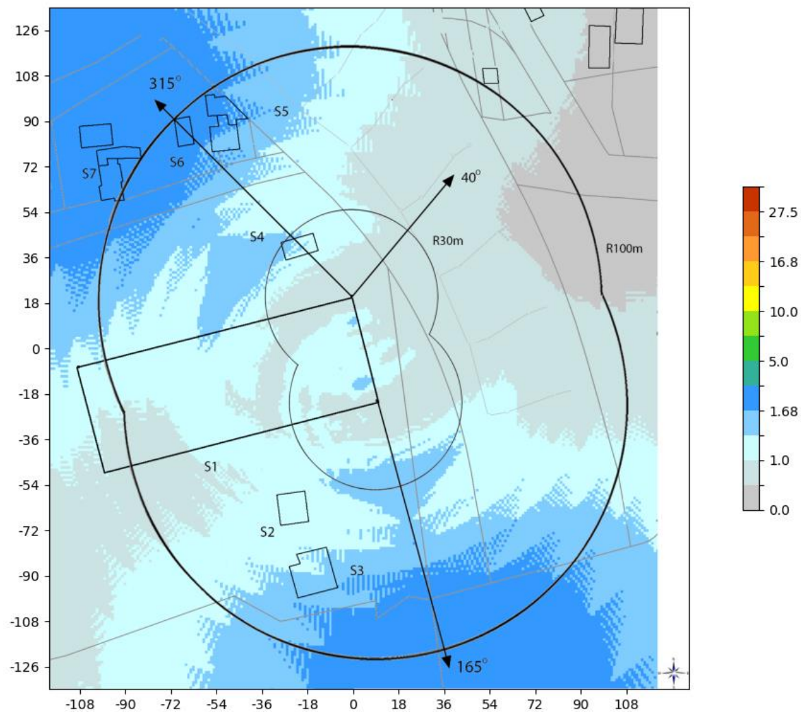
Slika 6.15. Rezultati proračuna jačine električnog polja na tlu, za slučaj kada sve stanice operatora MTS rade sa maks. kapacitetom.
