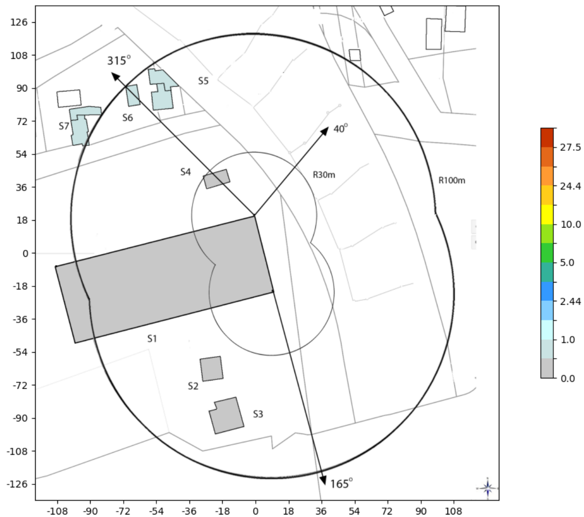
Slika 6.4. Rezultati proračuna jačine električnog polja unutar objekata, kada LTE2100 bazna stanica operatora MTS radi sa maks. kapacitetom.
