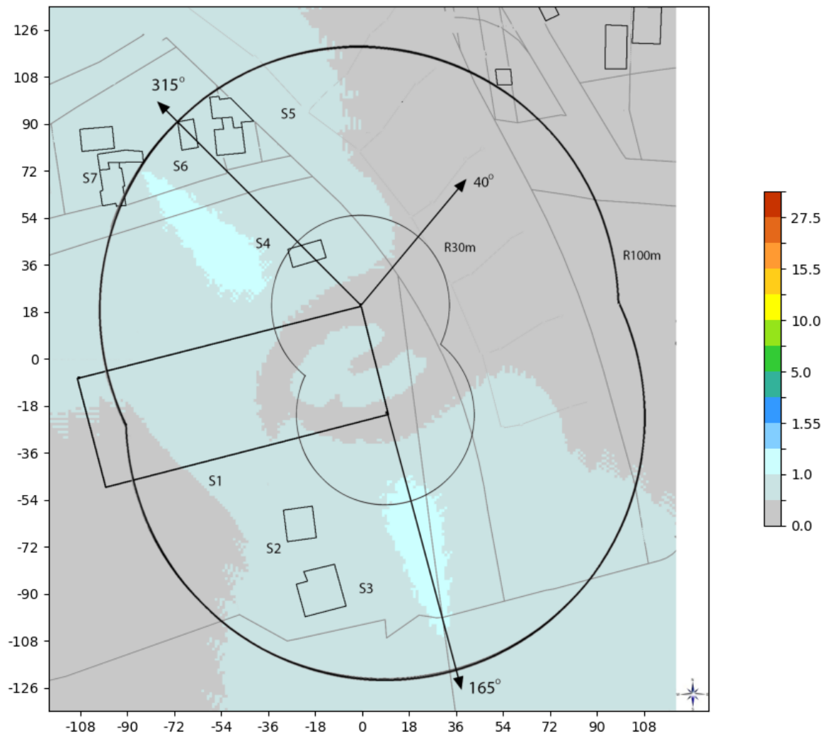
Slika 6.10. Rezultati proračuna jačine električnog polja na tlu, za slučaj kada LTE800 bazna stanica operatora MTS radi sa maks. kapacitetom.
