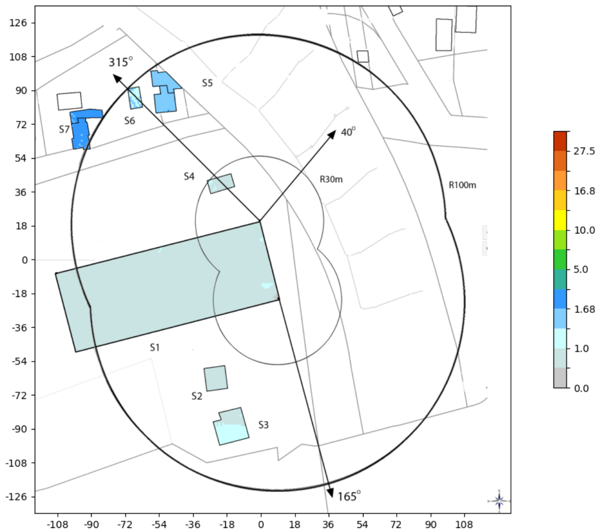
Slika 6.6. Rezultati proračuna jačine električnog polja unutar objekata, kada svi sistemi operatora MTS na lokaciji rade sa maksimalnim kapacitetom.
