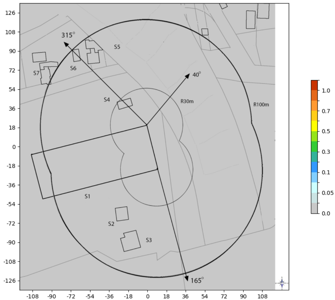
Slika 6.18: Rezultati proračuna faktora izlaganja na tlu, za slučaj kada svi sistemi svih operatera na lokaciji rade sa maksimalnim kapacitetom
