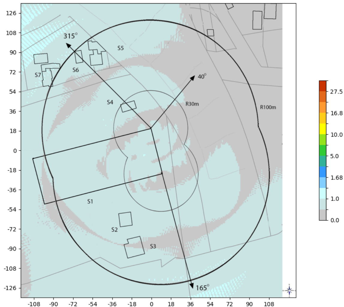
Slika 6.12. Rezultati proračuna jačine električnog polja na tlu, za slučaj kada GSM bazna stanica operatora MTS radi sa maks. kapacitetom.
