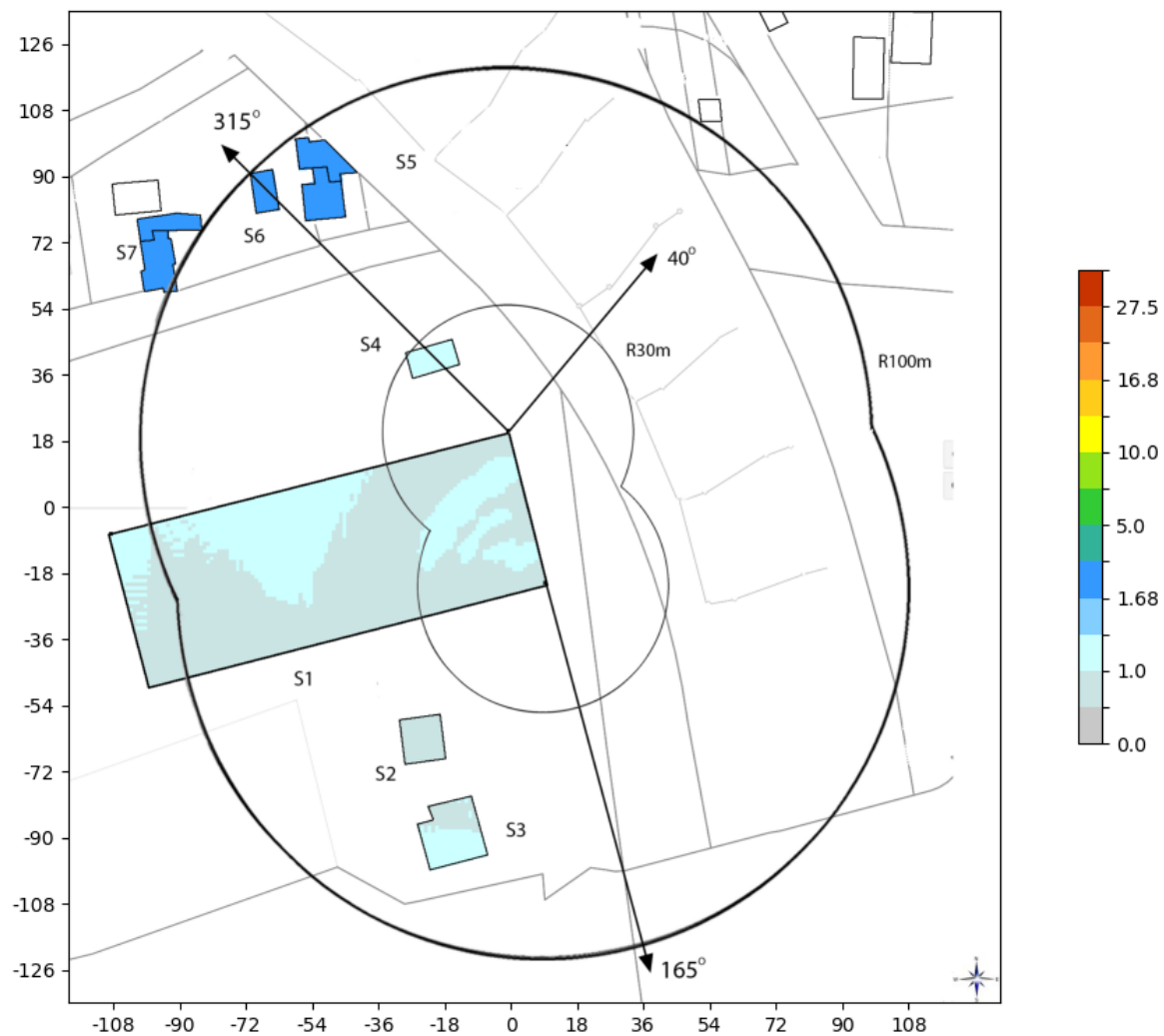
Slika 6.8. Rezultati proračuna jačine električnog polja unutar objekata, kada svi sistemi svih operatera rade sa maksimalnim kapacitetom.
