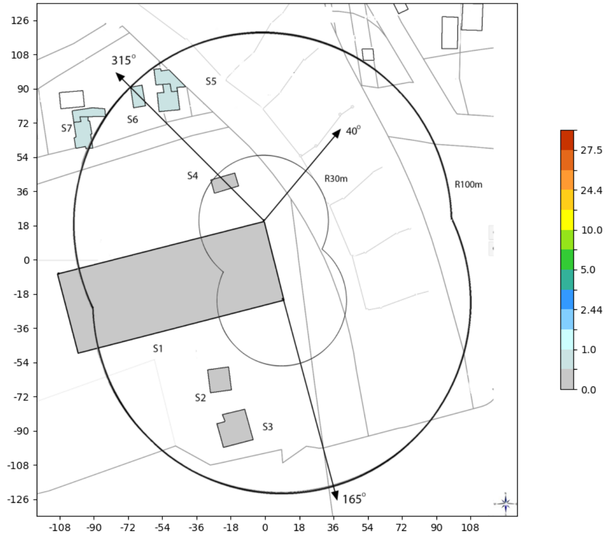
Slika 6.5. Rezultati proračuna jačine električnog polja unutar objekata, kada UMTS2100 bazna stanica operatora MTS radi sa maks. kapacitetom.
