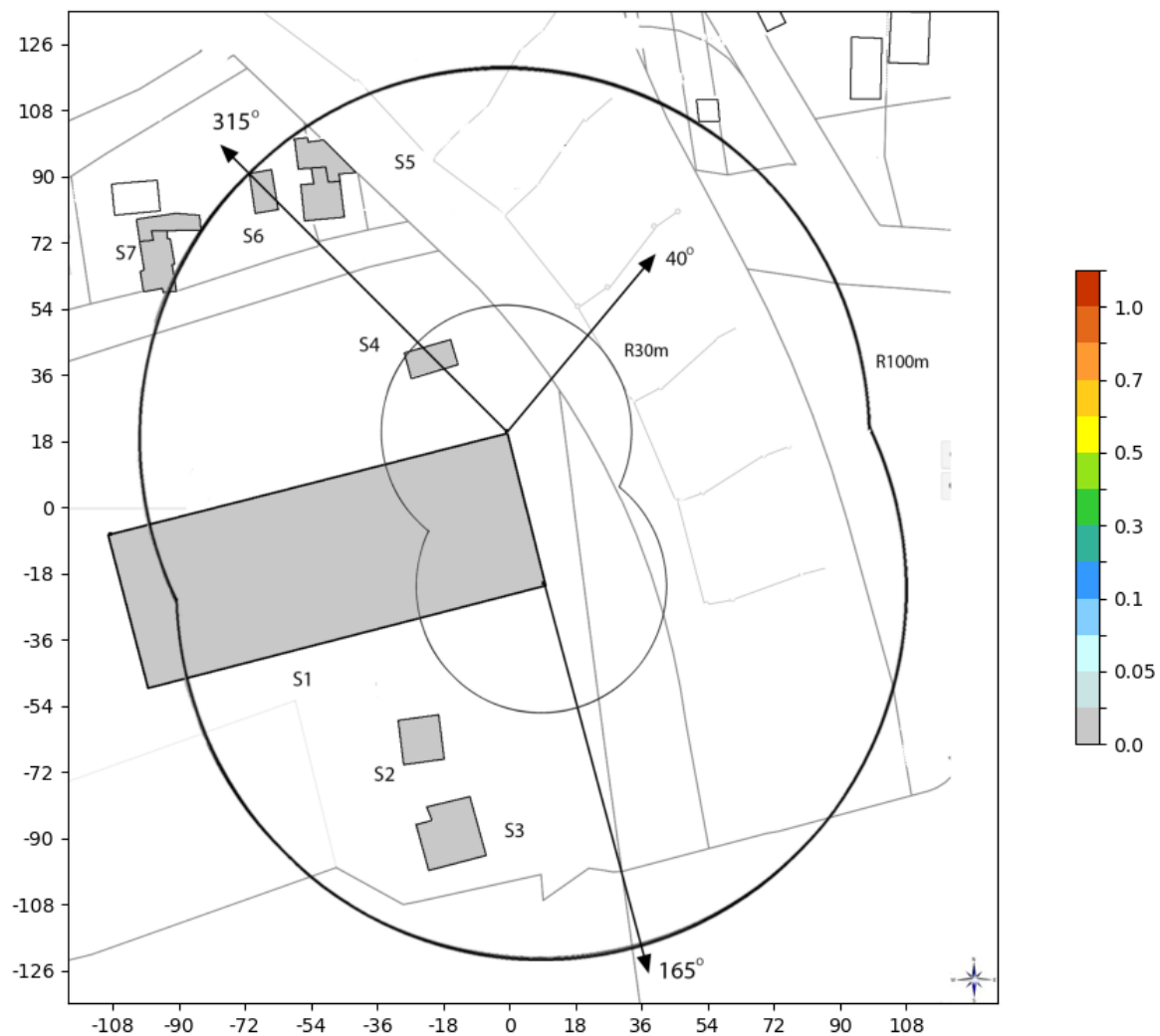
Slika 6.9. Rezultati proračuna faktora izlaganja unutar objekata, kada svi sistemi svih operatera rade sa maksimalnim kapacitetom.
