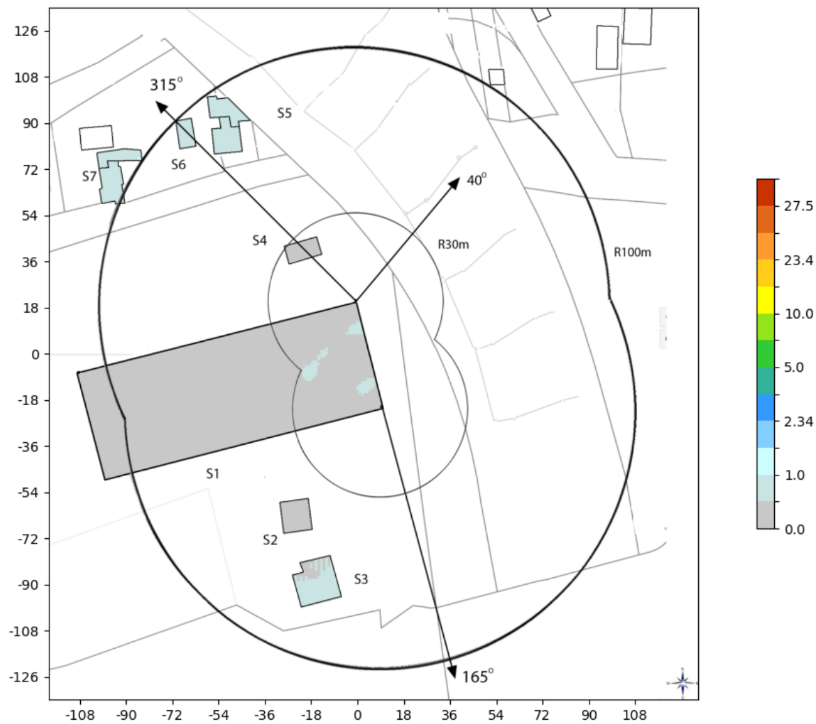
Slika 6.2: Rezultati proračuna jačine električnog polja unutar objekata, kada LTE1800 bazna stanica operatora MTS radi sa maksimalnim kapacitetom.
