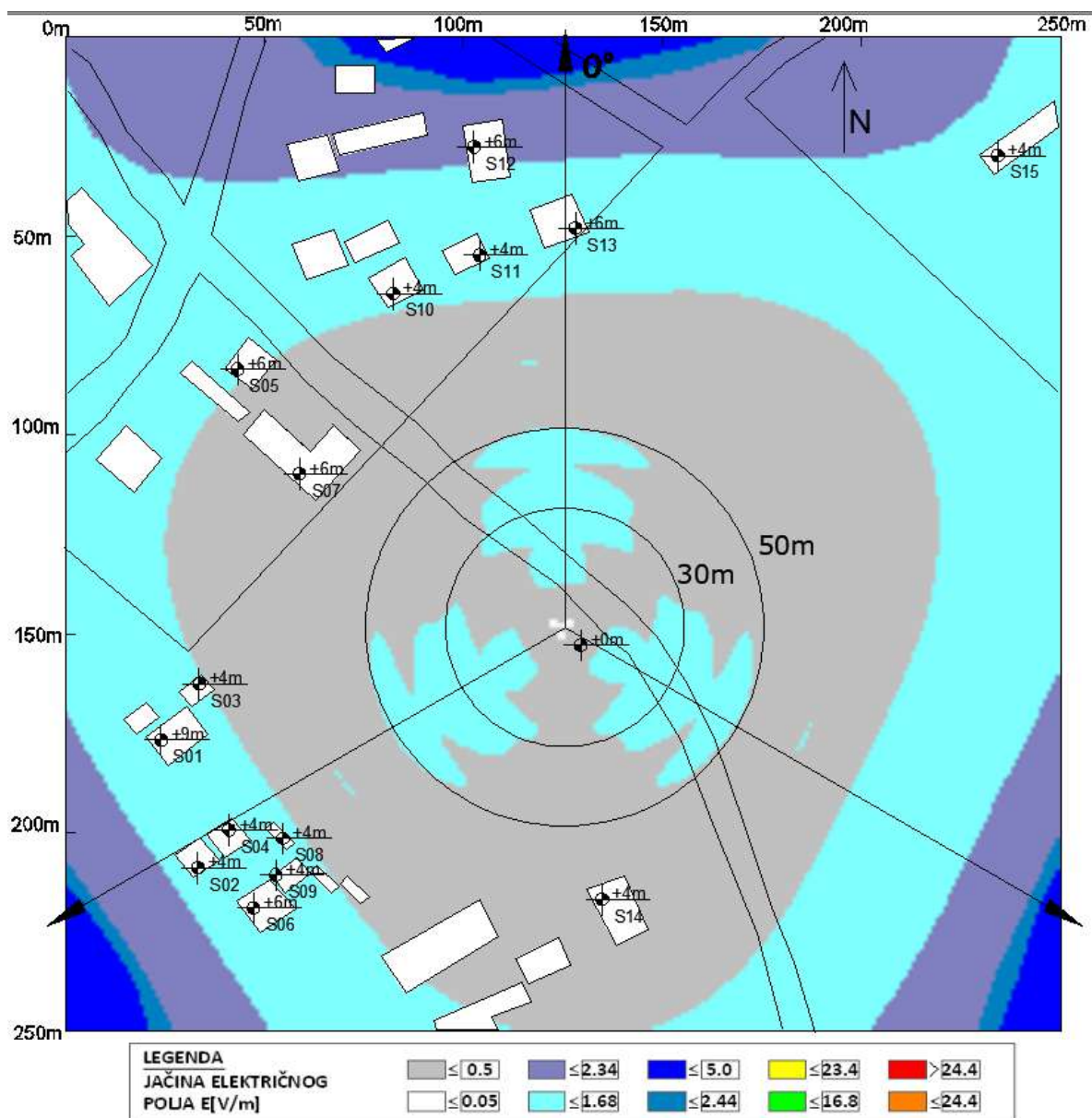
Slika 6.11 Rezultati proračuna jačine električnog polja u široj okolini lokacije bazne stanice na visini +1.70m (prosečna visina čoveka) u odnosu na nivo tla za slučaj rada svih sistema operatora A1 . Maksimalna proračunata vrednost jačine električnog polja iznosi E=2.71 V/m .
