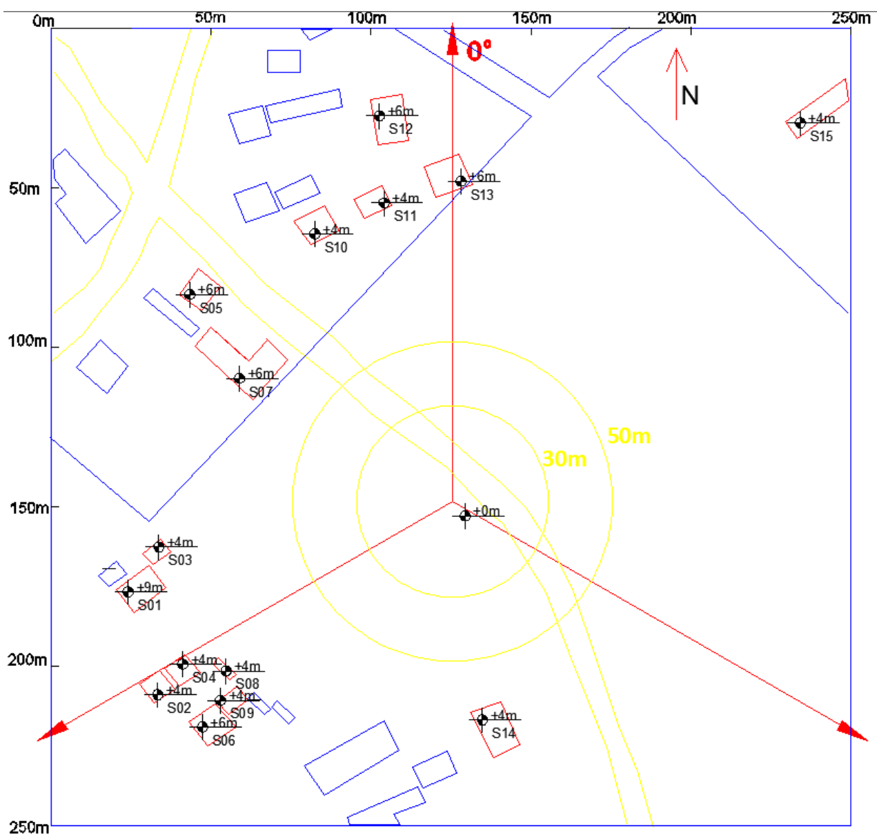
Slika 2.2 Dijagram objekata u okruženju radio bazne stanice „BG0371_01 BG_Obrenovac_Skela”
