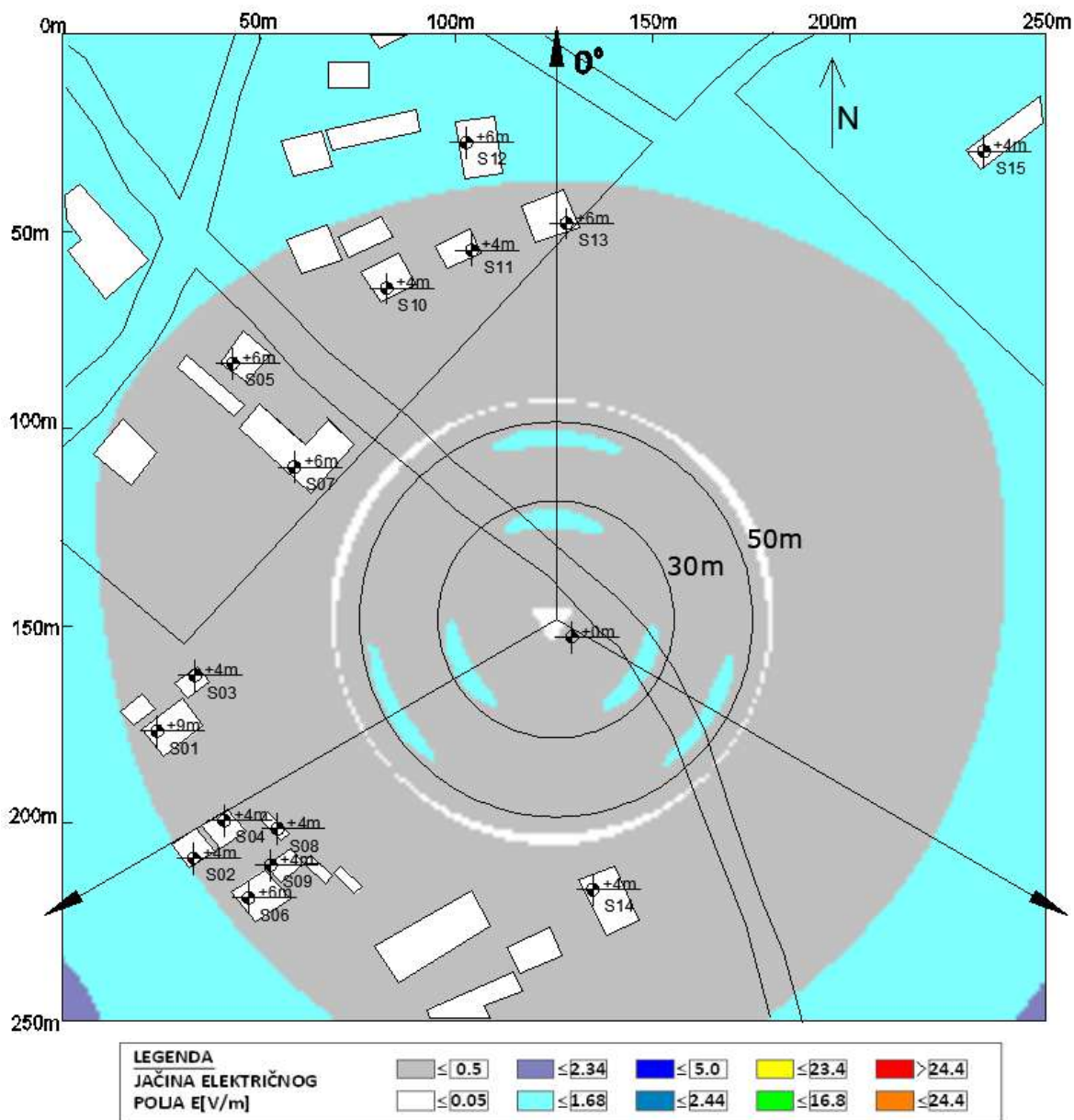
Slika 6.9 Maksimalna proračunata vrednost električnog polja na nivou tla u slučaju rada sistema LTE1800 operatora A1 Srbija iznosi: 1.76 V/m
