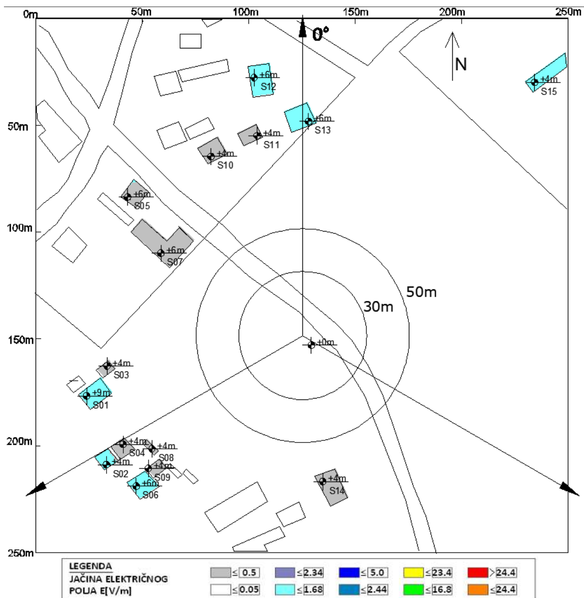
Slika 6.5 Rezultati proračuna jačine električnog polja u objektima na najizloženijim spratovima za slučaj rada svih sistema operatora A1
