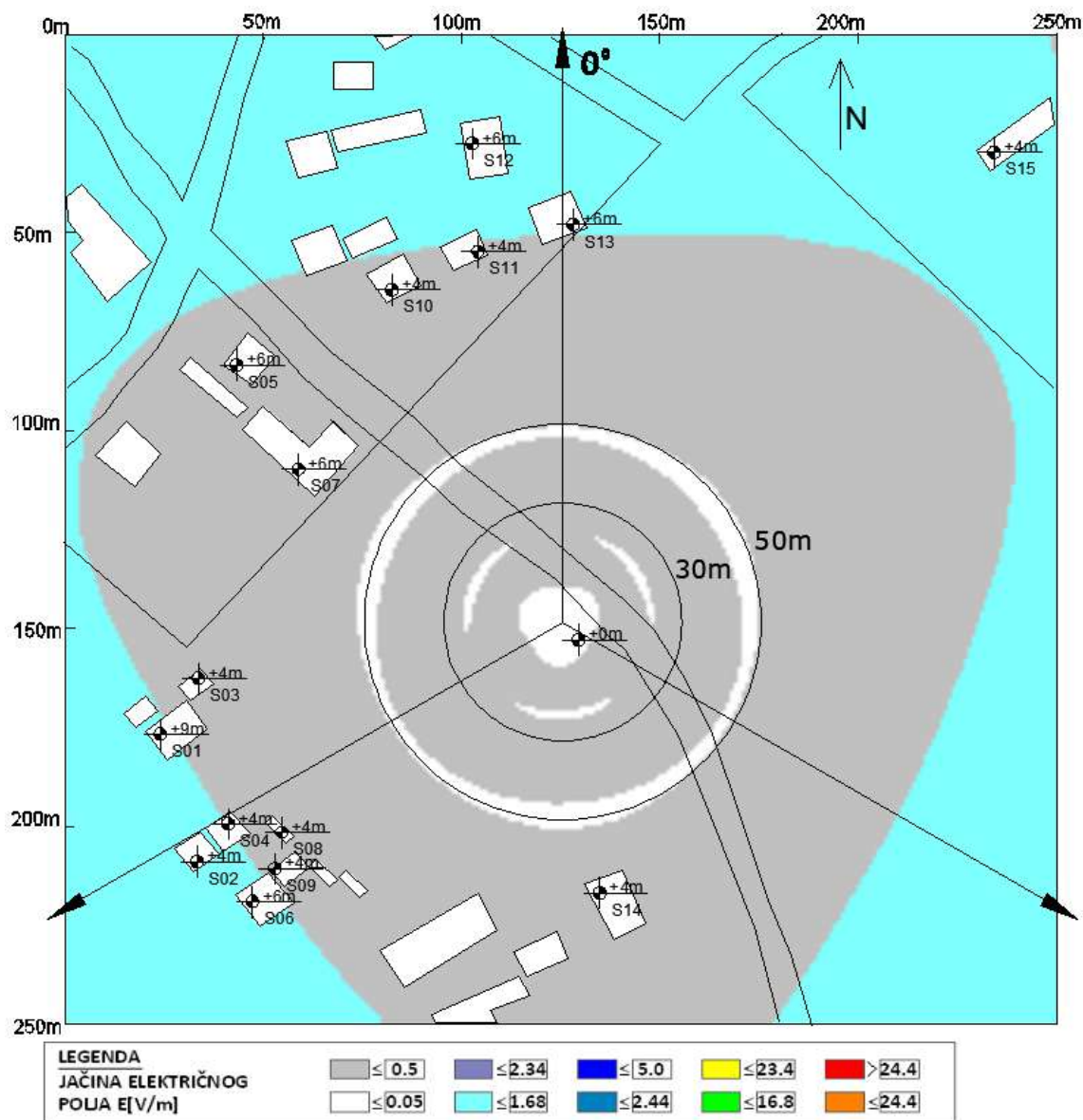
Slika 6.7 Maksimalna proračunata vrednost električnog polja na nivou tla u slučaju rada sistema GSM900 operatora A1 Srbija iznosi: 1.13 V/m
