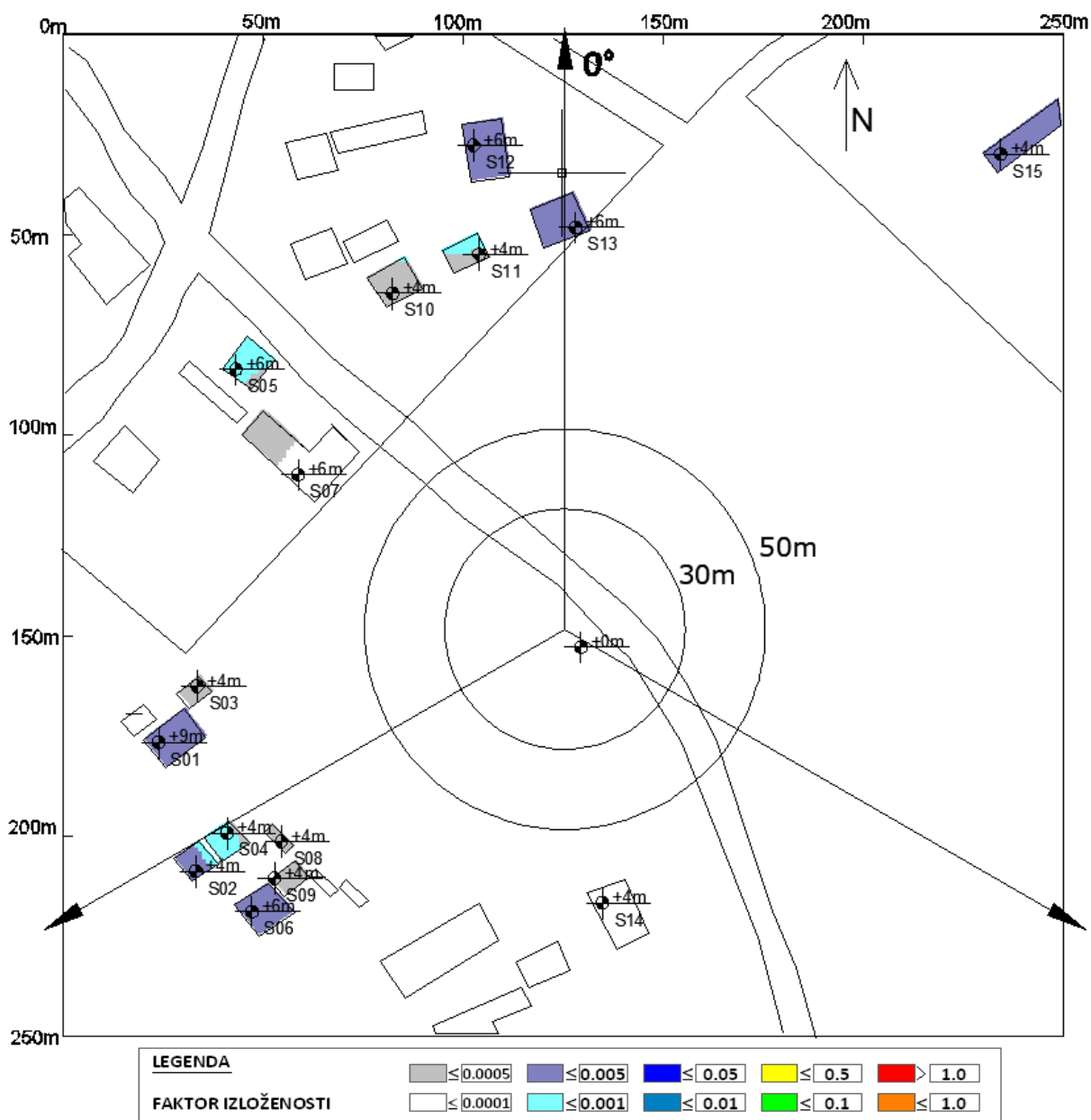
Slika 6.6 Rezultati proračuna faktora izloženosti u objektima na najizloženijim spratovima za slučaj rada svih sistema operatora A1
