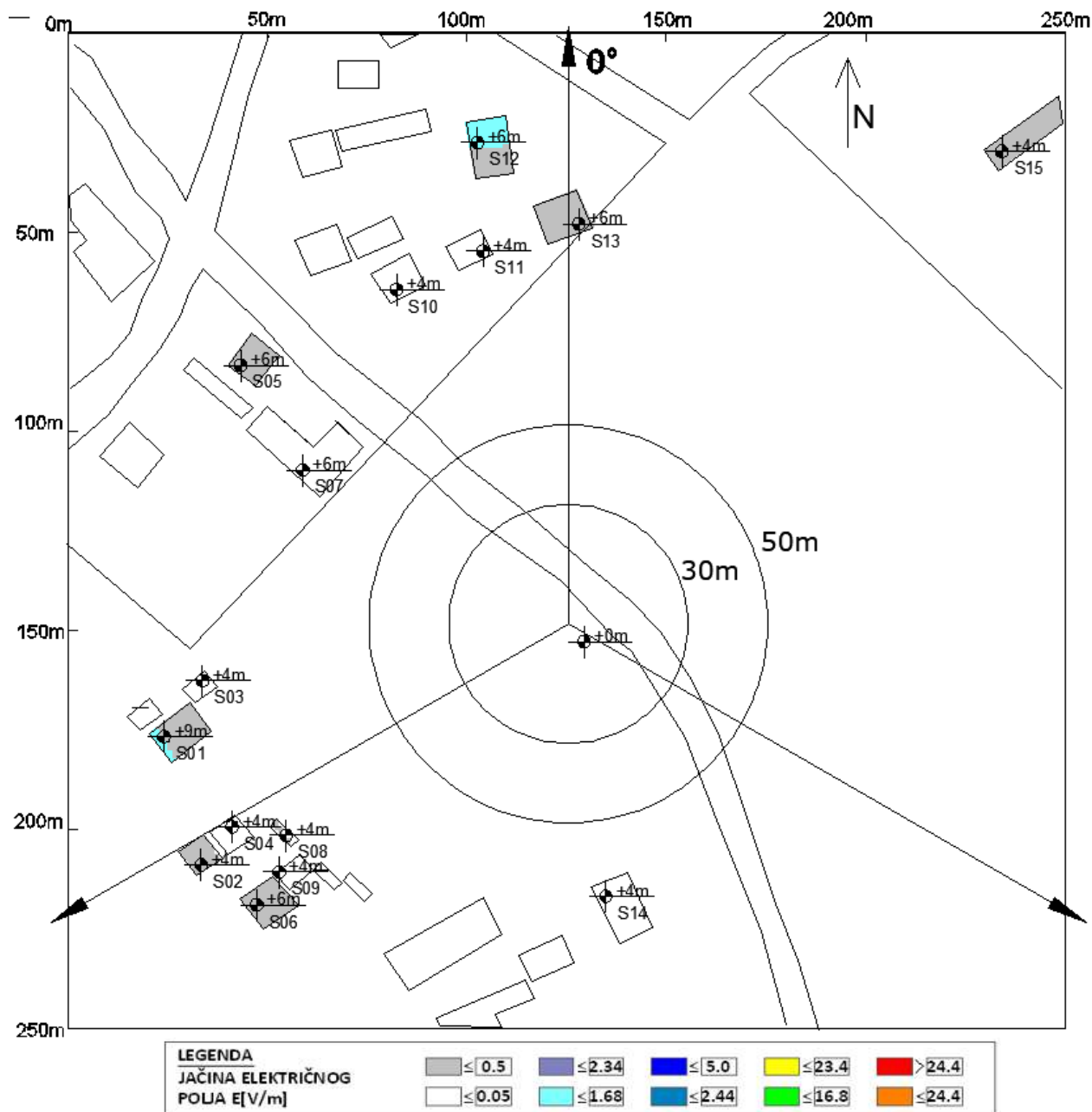
Slika 6.2 Rezultati proračuna jačine električnog polja u objektima na najizloženijim spratovima za slučaj rada sistema LTE2100 operatora A1 Srbija
