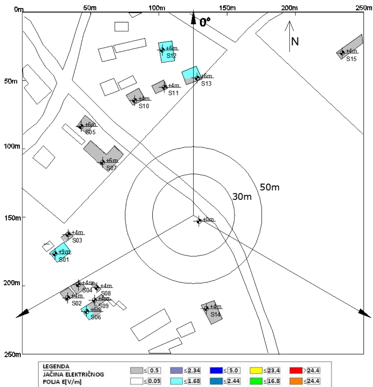
Slika 6.4 Rezultati proračuna jačine električnog polja u objektima na najizloženijim spratovima za slučaj rada sistema LTE800 operatora A1 Srbija
