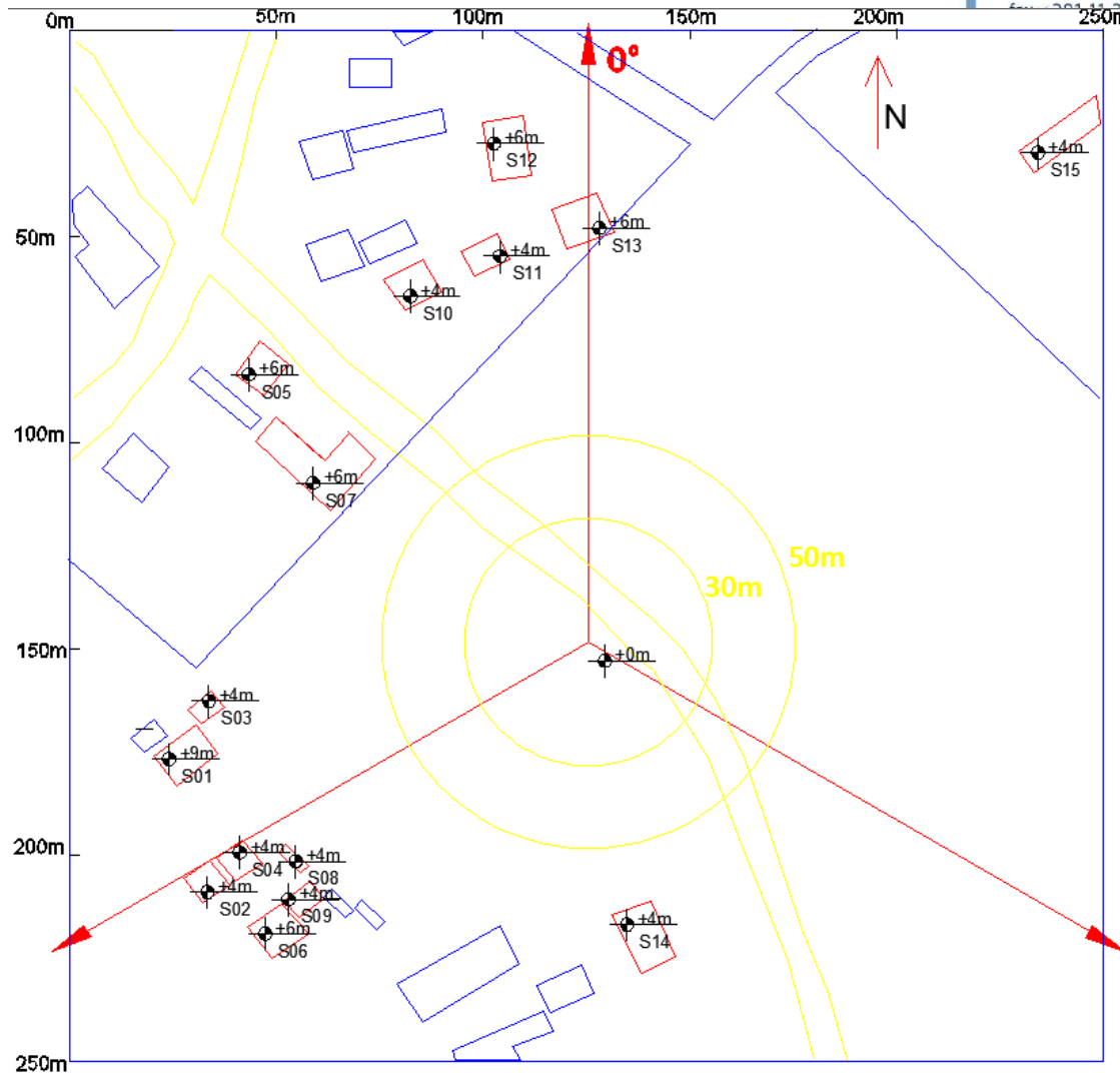
Slika 5.2. Dijagram objekata u okruženju bazne stanice „BG0371_01 BG_Obrenovac_Skela”
