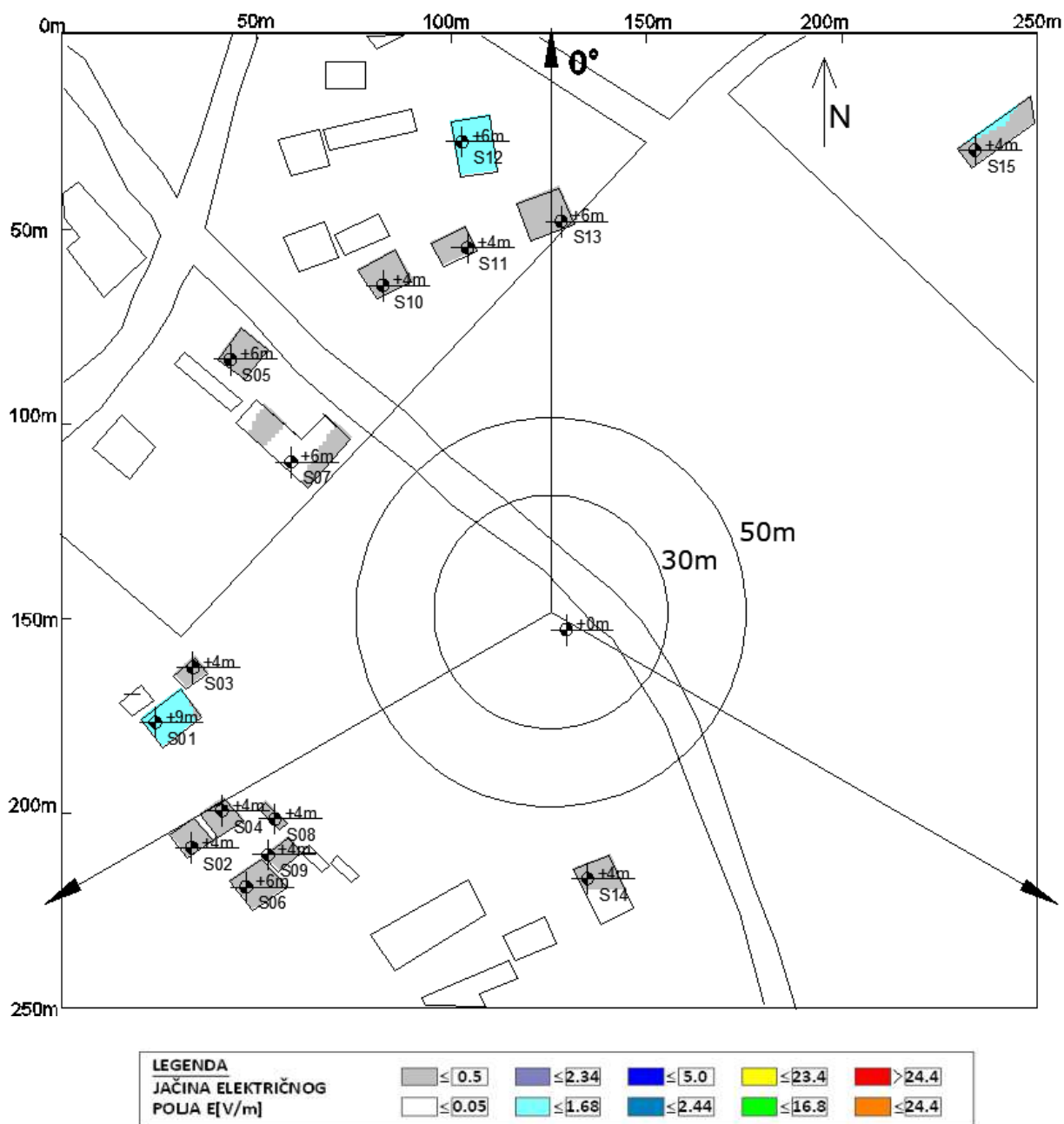
Slika 6.3 Rezultati proračuna jačine električnog polja u objektima na najizloženijim spratovima za slučaj rada sistema LTE1800 operatora A1 Srbija
