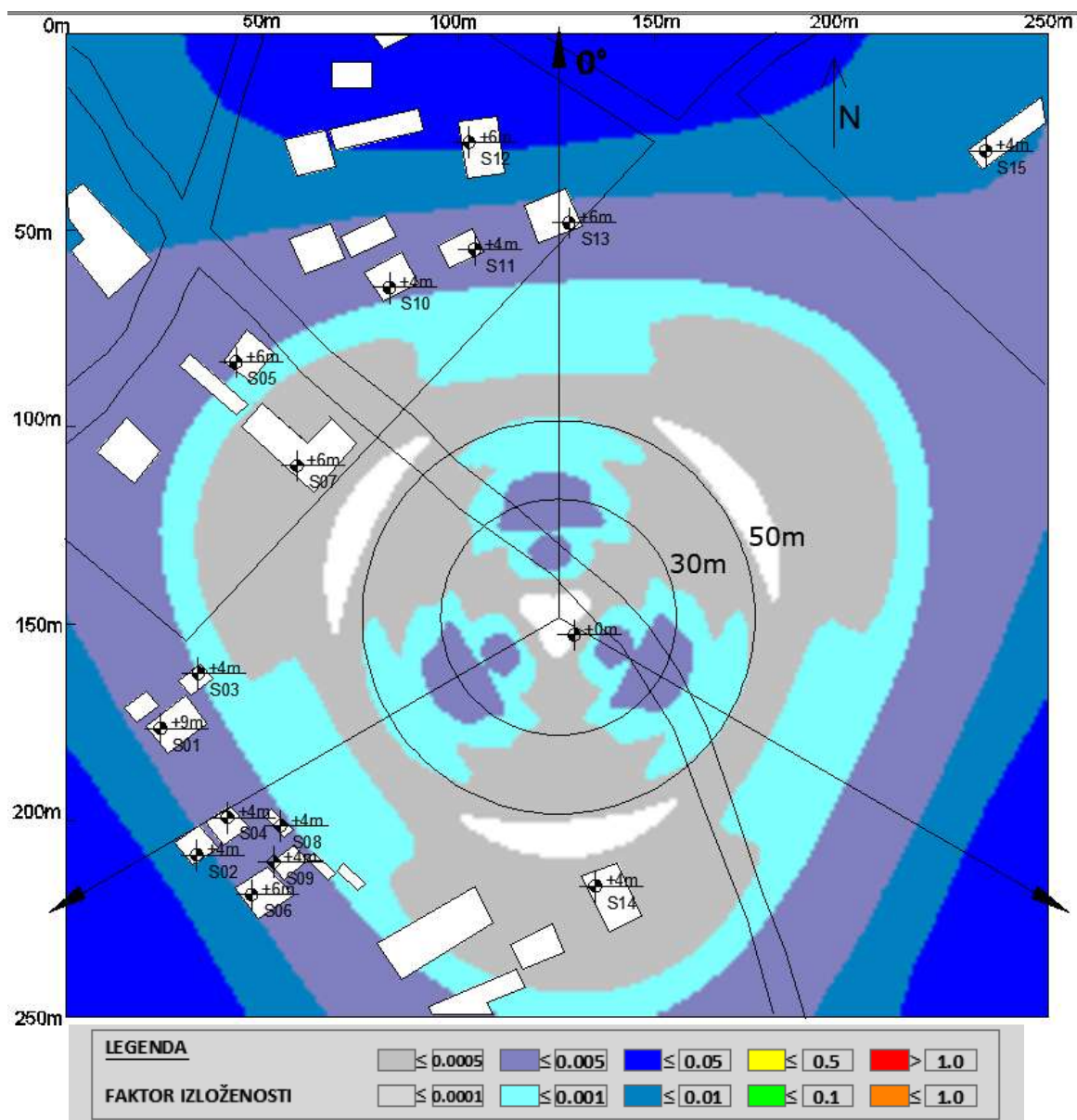
Slika 6.12 Rezultati proračuna faktora izloženosti u široj okolini lokacije bazne stanice na visini +1.70m (prosečna visina čoveka) u odnosu na nivo tla za slučaj rada svih sistema operatora A1 . Maksimalna proračunata vrednost faktora izloženosti iznosi FI=0,0188 .
