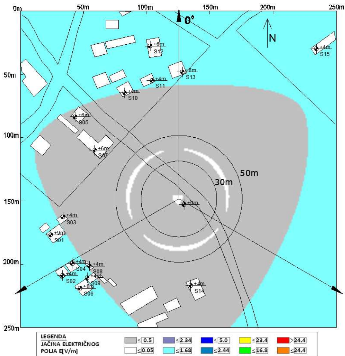
Slika 6.10 Maksimalna proračunata vrednost jačine električnog polja na nivou tla u slučaju rada sistema LTE800 na predmetnoj lokaciji operatora A1 Srbija iznosi: 1.23 V/m
