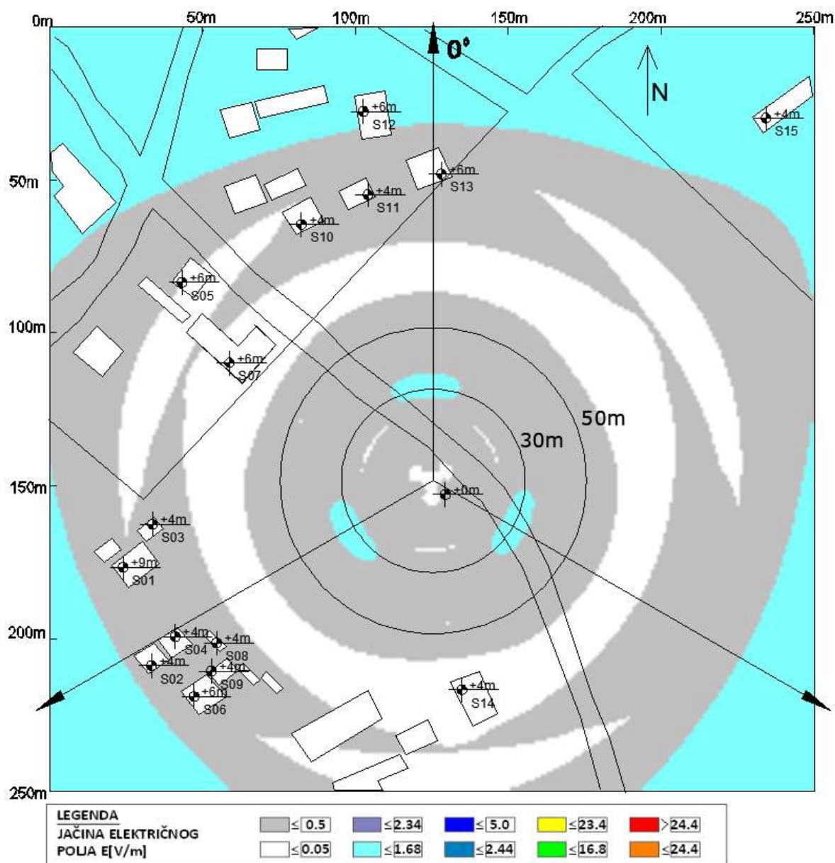
Slika 6.8 Maksimalna proračunata vrednost električnog polja na nivou tla u slučaju rada sistema LTE2100 operatora A1 Srbija iznosi: 1.26 V/m
