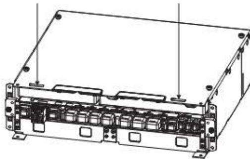
Slika.2 Izgled Flexi Multiradio 10 BTS sistemskog modula
