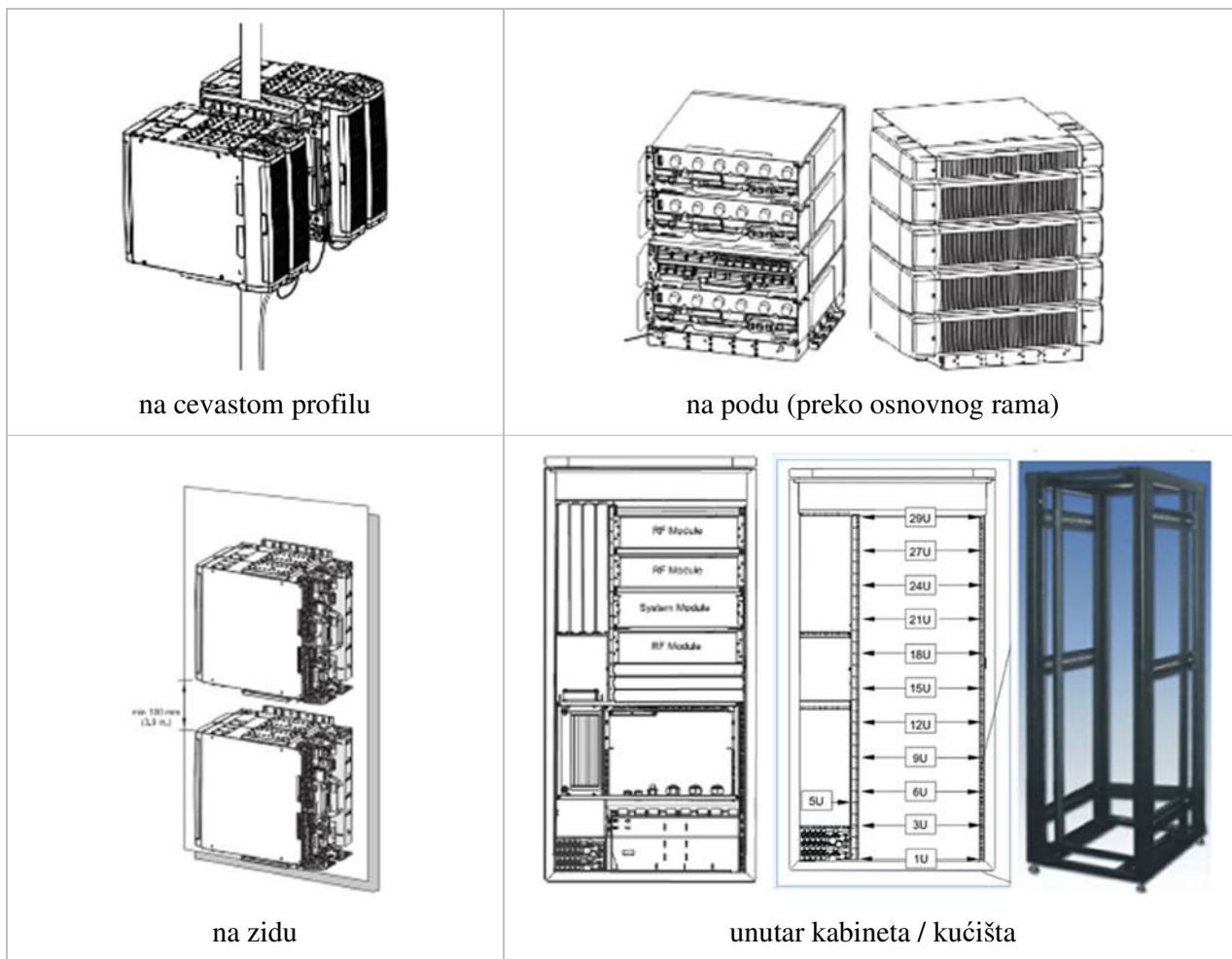
Slika.4 Mogući scenariji montaže Flexi modula
