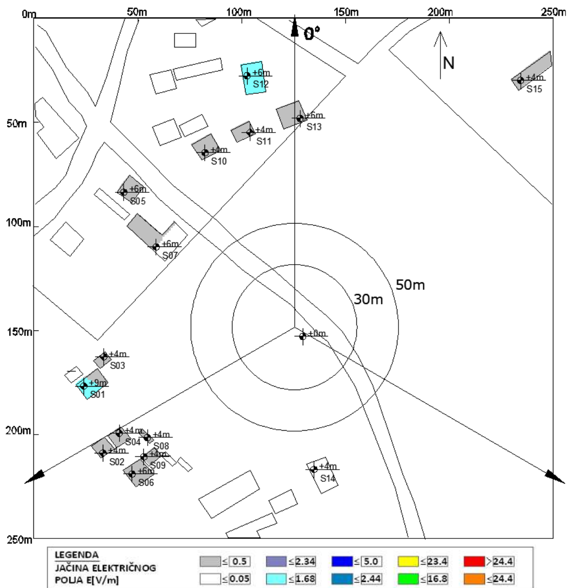
Slika 6.1 Rezultati proračuna jačine električnog polja u objektima na najizloženijim spratovima za slučaj rada sistema GSM900 operatora A1 Srbija
