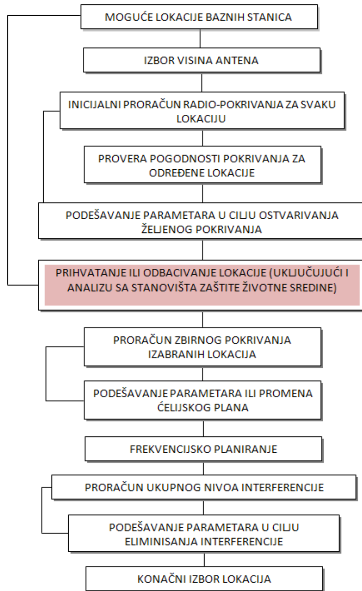
Slika.1 Procedura izbora mikrolokacija baznih stanica
