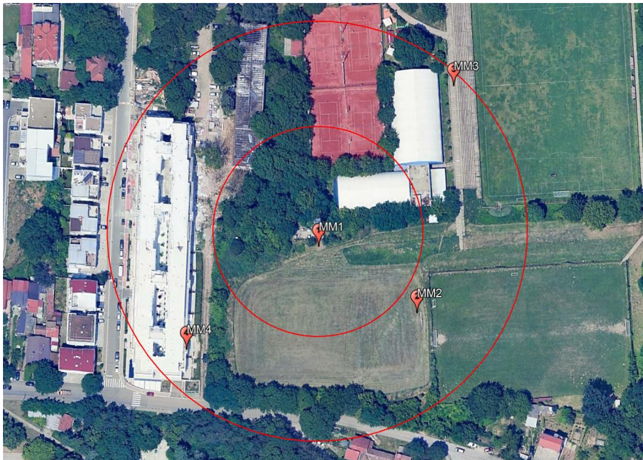
Slika 6: Prikaz Mernih Mesta u lokalnoj zoni FM radio stanice Radio Lola 106.3
