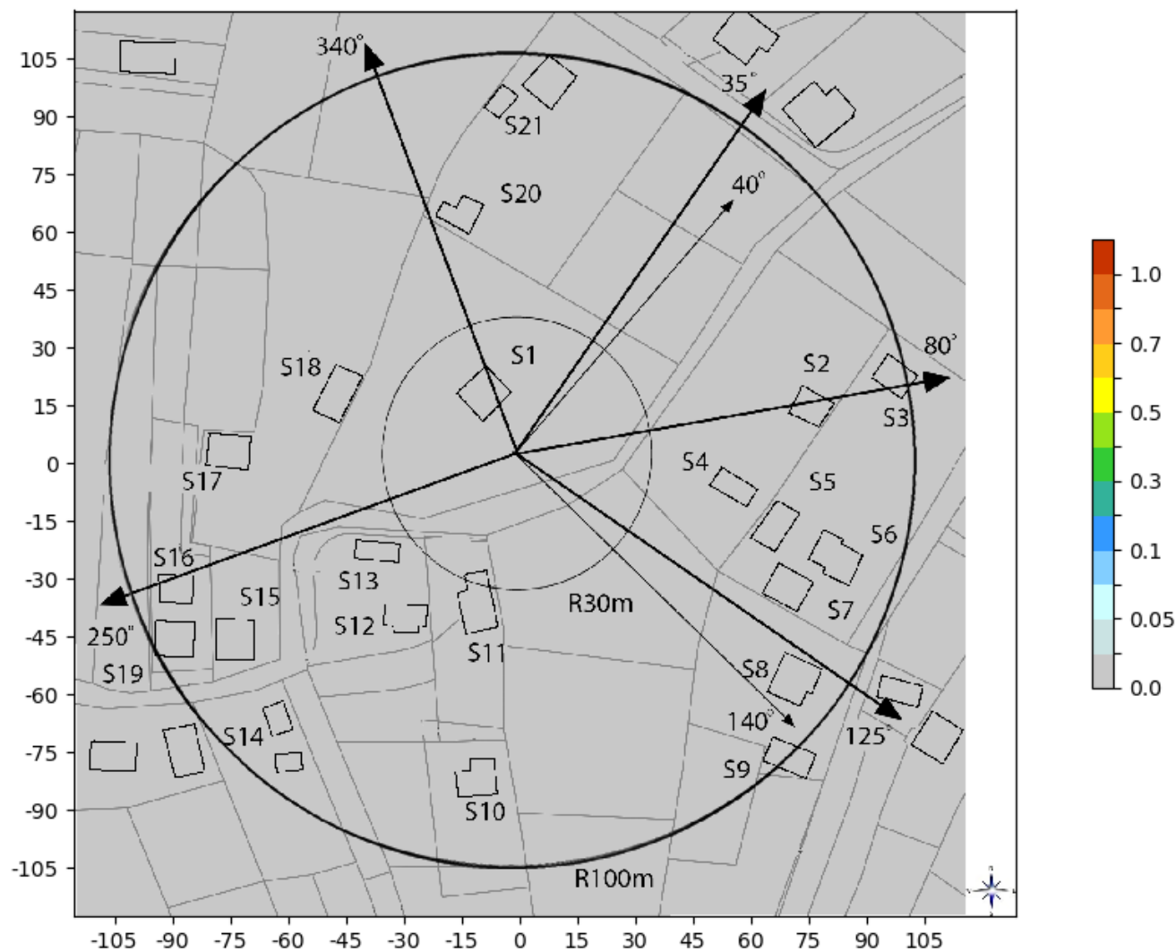
Slika 6.18: Rezultati proračuna faktora izlaganja na tlu, za slučaj kada svi sistemi svih operatora na lokaciji rade sa maksimalnim kapacitetom
