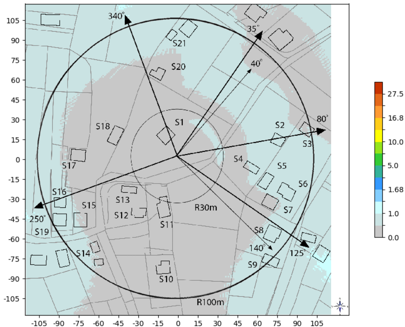
Slika 6.12. Rezultati proračuna jačine električnog polja na tlu, za slučaj kada GSM bazna stanica operatora MTS radi sa maks. kapacitetom.
