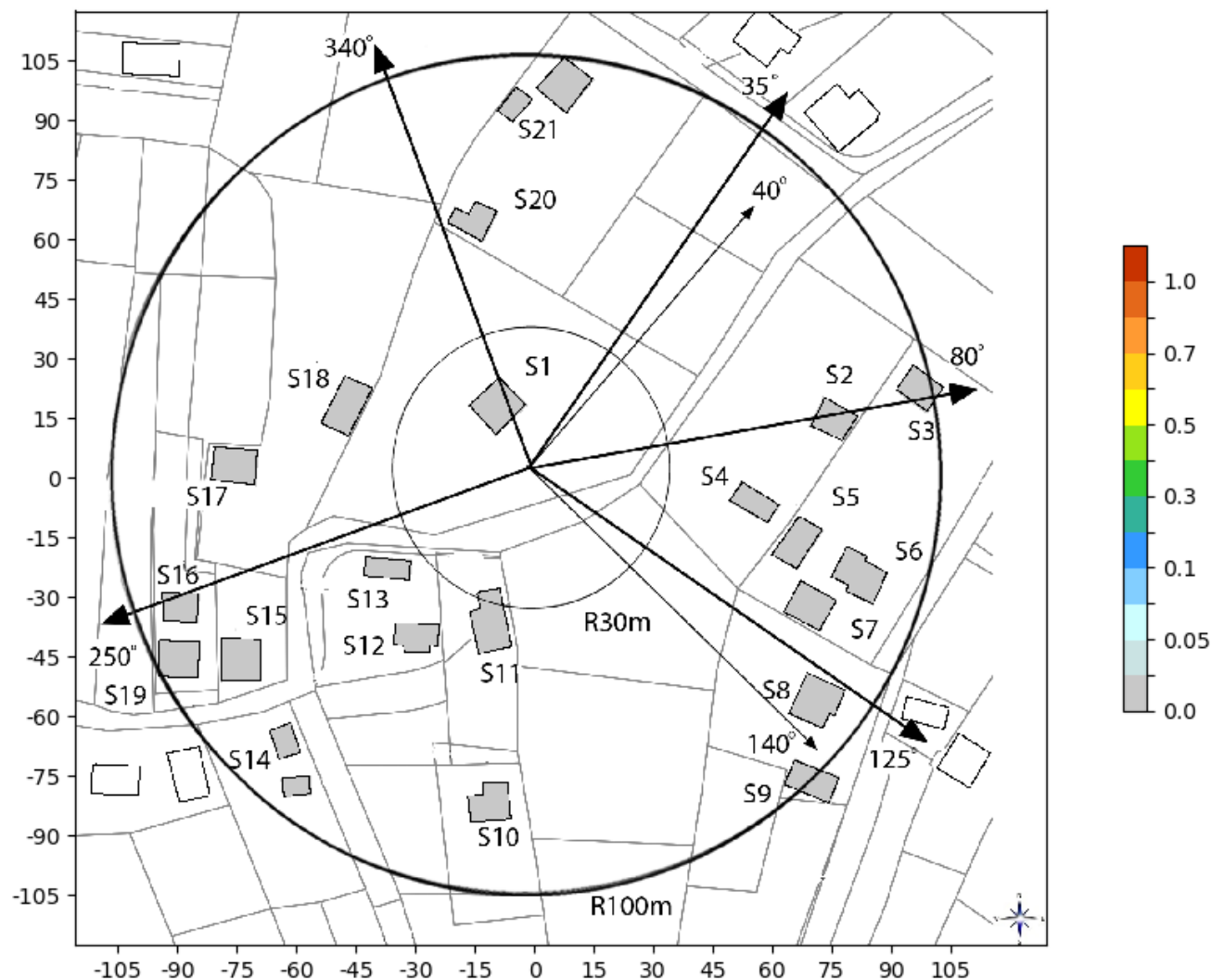
Slika 6.9. Rezultati proračuna faktora izlaganja unutar objekata, kada svi sistemi svih operatora rade sa maksimalnim kapacitetom.
