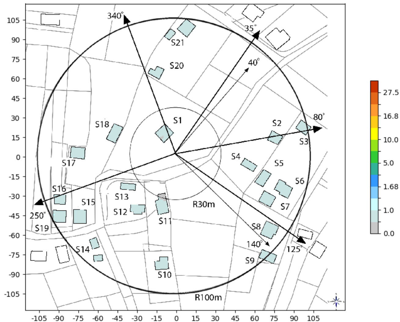
Slika 6.8. Rezultati proračuna jačine električnog polja unutar objekata, kada svi sistemi svih operatora rade sa maksimalnim kapacitetom.
